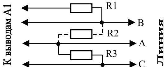
Рисунок 3 – Схема «перекоса» входа приемников
