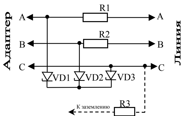
Рисунок 4 – Схема защиты от перенапряжений
