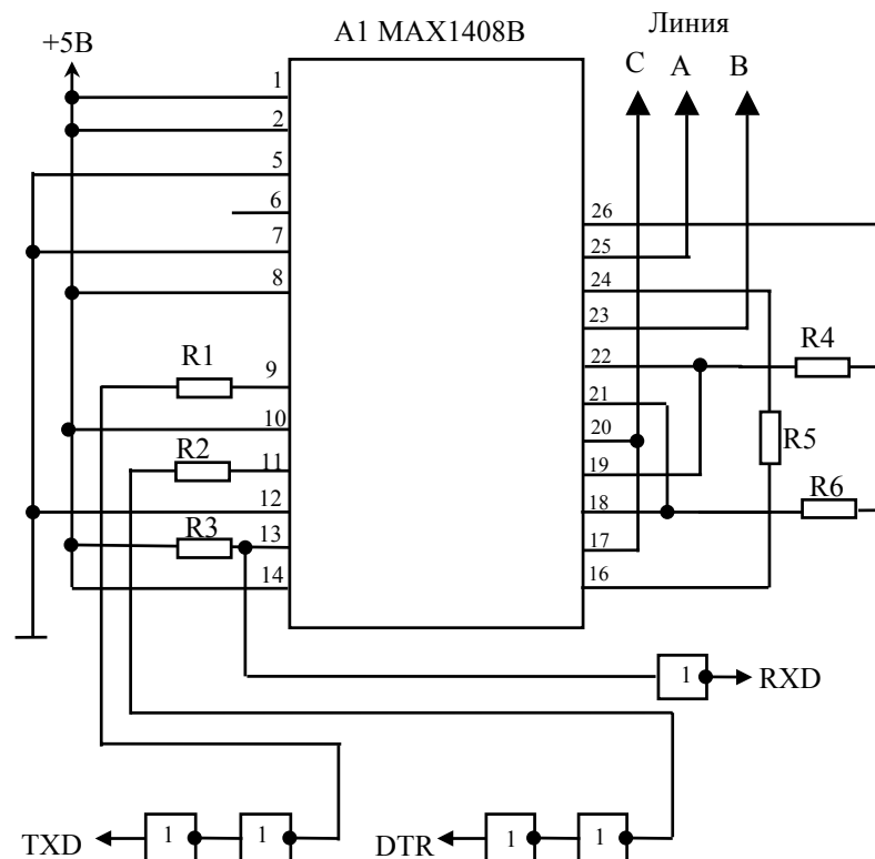
Рисунок 2 – Принципиальная электрическая схема адаптера АП
