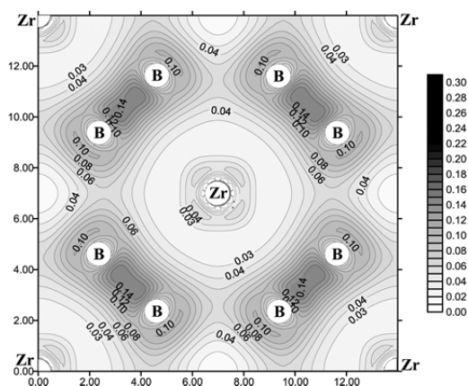
Рис. 5. Распределение электронной плотности в плоскости (001), проходящей через пять Zr и восемь В атомов. Здесь и на рис. 6 расстояния даны в а.е.д., а плотность заряда в e/(\text{а.е.д.})^3 , где e — элементарный электрический заряд.
