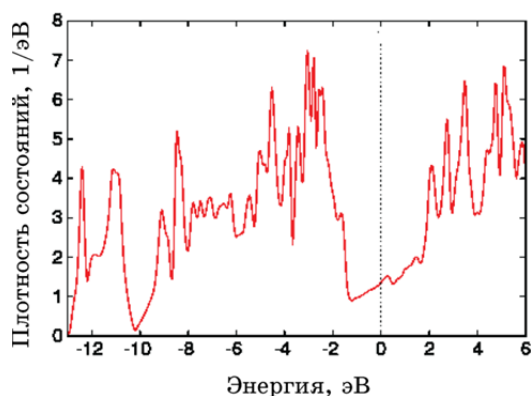
Рис. 3. Полная плотность электронных состояний в додекабориде циркония.
