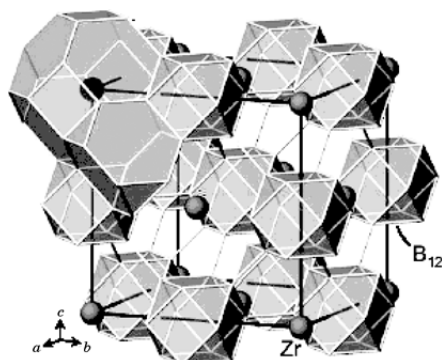
Рис. 1. Кристаллическая структура додекаборида циркония — симметрия Fm\bar{3}m , параметр решетки при комнатной температуре a = 7,4072 \pm 0,0005 Å, объем элементарной ячейки V = 406,5 Å 3 , расстояние между ближайшими атомами бора — от 1,68 Å до 1,78 Å [12].
