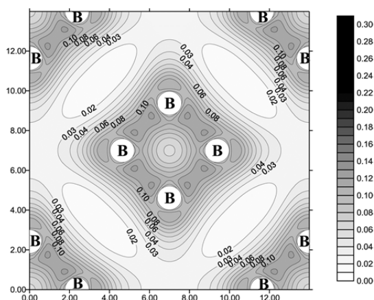
Рис. 6. Распределение электронной плотности в плоскости (001), проходящей через шестнадцать В атомов.
