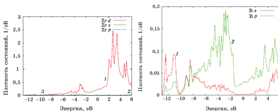
Рис. 4. Парциальные плотности электронных состояний подрешеток циркония и бора в ZrB_{12} . Цифрами 1, 2, 3 указаны состояния s , p , d .
