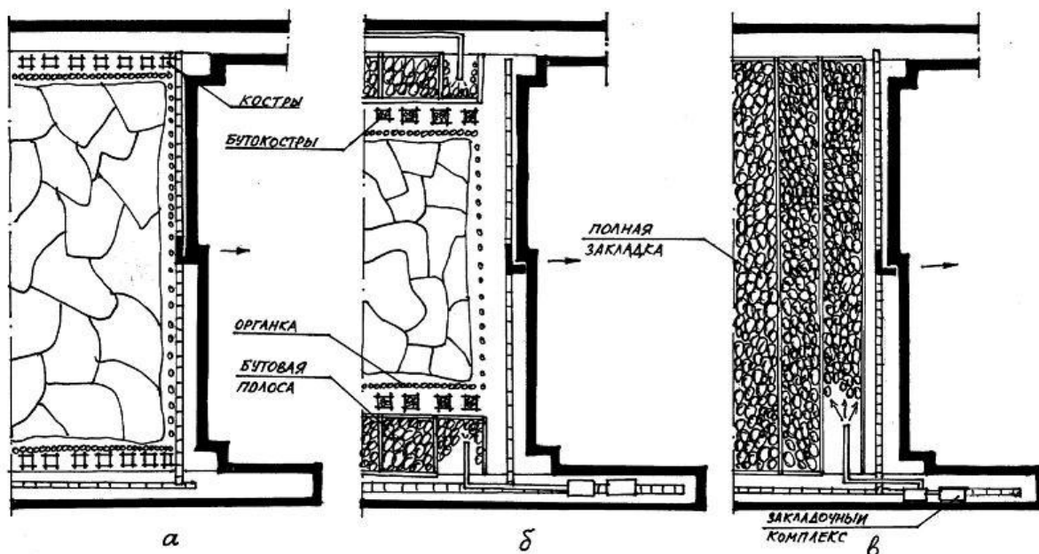
Рисунок 4 – Технологические схемы крепления в очистном забое:
