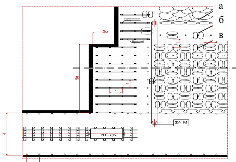
Рисунок 5 – Технологическая схема крепления с использованием:
