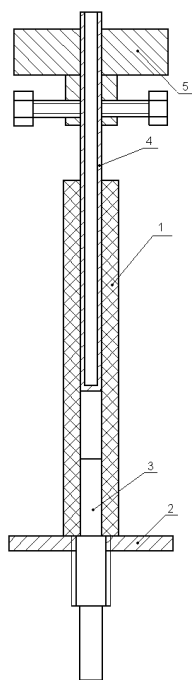
Рис. 1. Прибор для измерения электрического сопротивления угля
