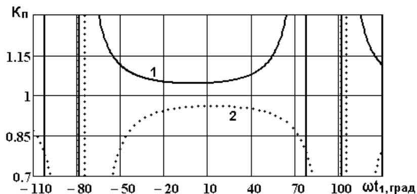
Рисунок 3 – Зависимость коэффициента погрешности k_n от момента первого отсчета \omega t_1 при поперечной несимметрии: 1) k_{нс} = 0,5 ; 2) k_{нс} = 1,5 . Утечка в фазе С
