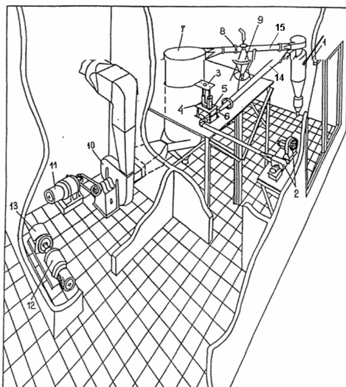
Рис. 2 – Загальний вигляд експериментального стенду.
