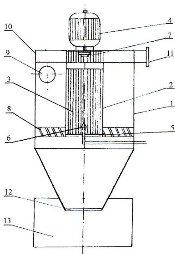
Рис. 1. Пиловловлювач
