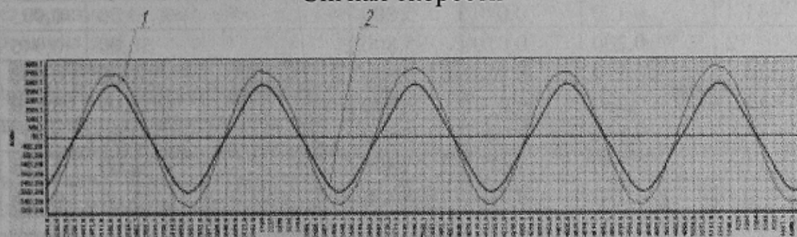
Сигнал перемещения
