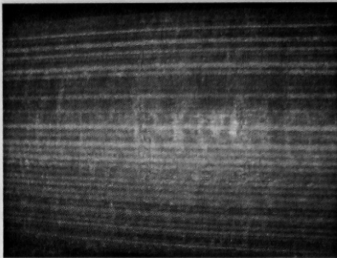
Рисунок 2 - Надрывы, складчатость и поперечные трещины на поверхности чернового слитка
