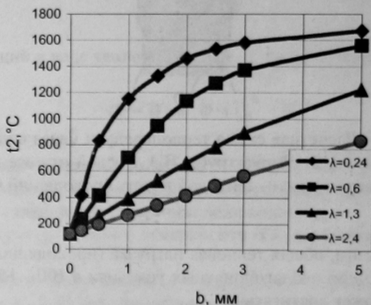
Рисунок 2 – Зависимость температуры рабочей поверхности ВЭ ( t_2 ) от толщины отложений на охлаждаемой поверхности ( b ) и их теплопроводности ( \lambda , Вт/(м·К)).
