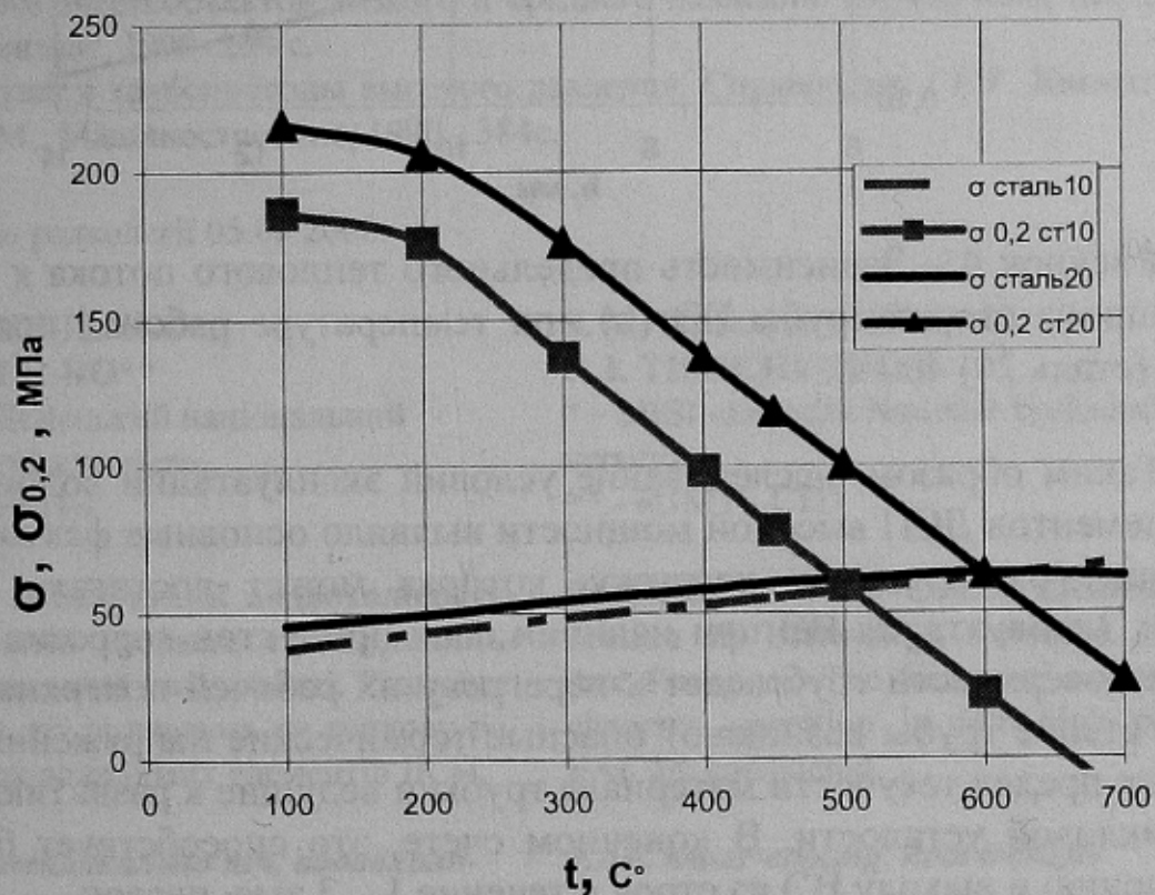
Рисунок 3 – Зависимость предела текучести \sigma_{0,2} (линии с маркерами) и возникающих в стенке трубы напряжений (линии без маркеров) от температуры поверхности трубы для материалов: сталь 10 и сталь 20.
