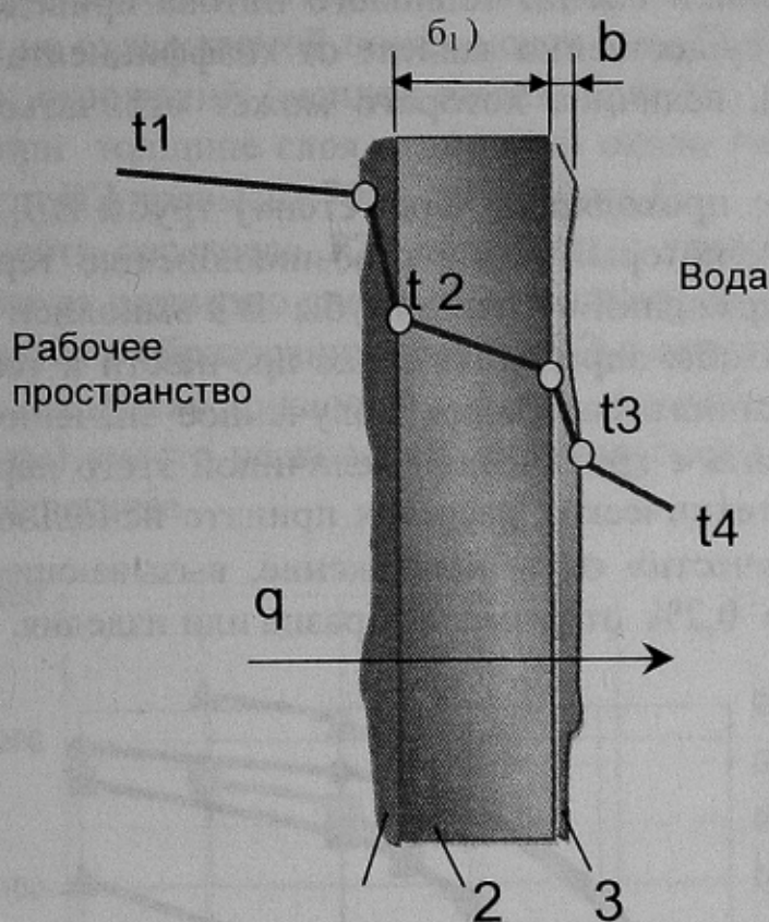
Рисунок 1 – Расчетная схема теплопередачи через водоохлаждаемый элемент. 1- гарнисаж, 2- стенка трубы ВЭ, 3- слой отложений на охлаждаемой водой поверхности, q - тепловой поток, проходящий к воде.
