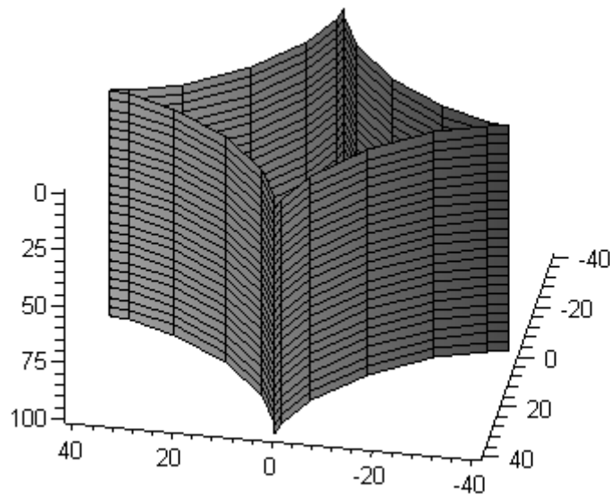
Рис.2 Астроїдальна циліндрична поверхня
