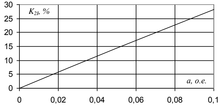
Рисунок 2 – Обобщенная зависимость коэффициента ОП по току K_{2I} от количества замкнувшихся витков обмотки статора АД a
