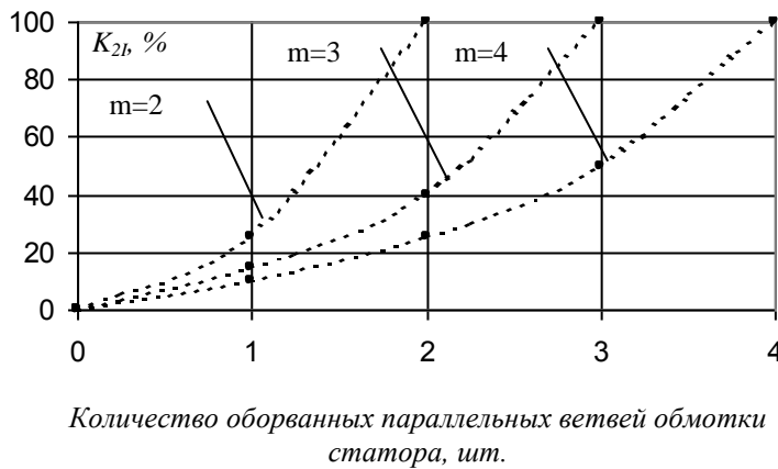
Рисунок 3 – Обобщенные зависимости коэффициента ОП по току K_{2l} от количества оборванных параллельных ветвей обмотки статора АД
