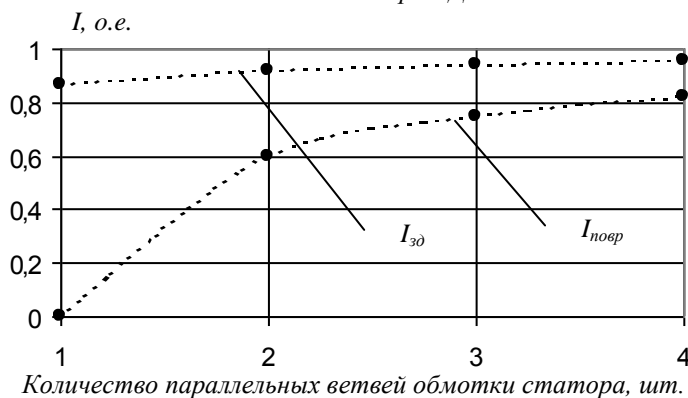
Рисунок 4 – Зависимости токов в «здоровых» I_{3д} и поврежденной I_{повр} фазах от количества параллельных ветвей обмотки статора при обрыве одной из этих ветвей в одной фазе
