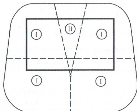
Рис. 7. Зоны деформаций в мульдe сдвигения при неполной подработке вкрест простирания; при полной подработке по простиранию со стороны восстания и при неполной подработке по простиранию со стороны падения
