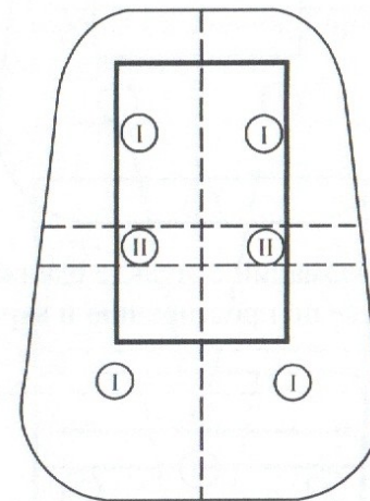
Рис. 5. Зони деформацій в мульдї сдвигнення при неповній подроботці по простиранию і повній подроботці вкрест простиранию
