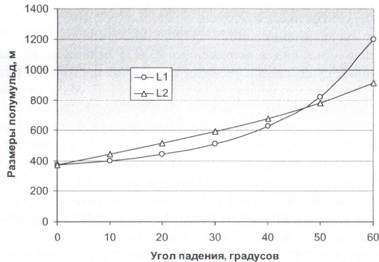
Рис. 1. Динамика изменения размеров полумульд по падению и востанню при увеличении угла падения пласта
