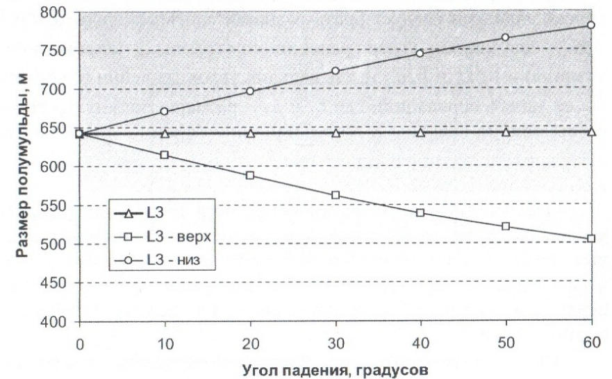
Рис. 2. Динамика изменения размеров полумульды по простиранию при увеличении угла падения пласта
