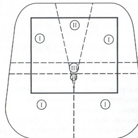
Рис. 8. Зоны деформаций в мульдe сдвигения при полной подработке вкрест простирания; при полной подработке по простиранию со стороны восстания и при неполной подработке по простиранию со стороны падения
