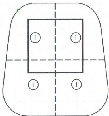
Рис. 6. Зони деформаций в мульдe сдвигения при неполной подработке по простиранию и вкрест простирания
