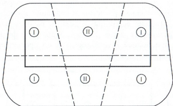
Рис. 4. Зони деформацій в мульдї сдвигнення при повній подроботці по простиранию і неповній подроботці вкрест простиранию
