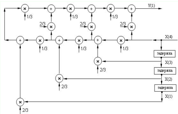
Рисунок 1. – Схема реализации алгоритма, m=4
