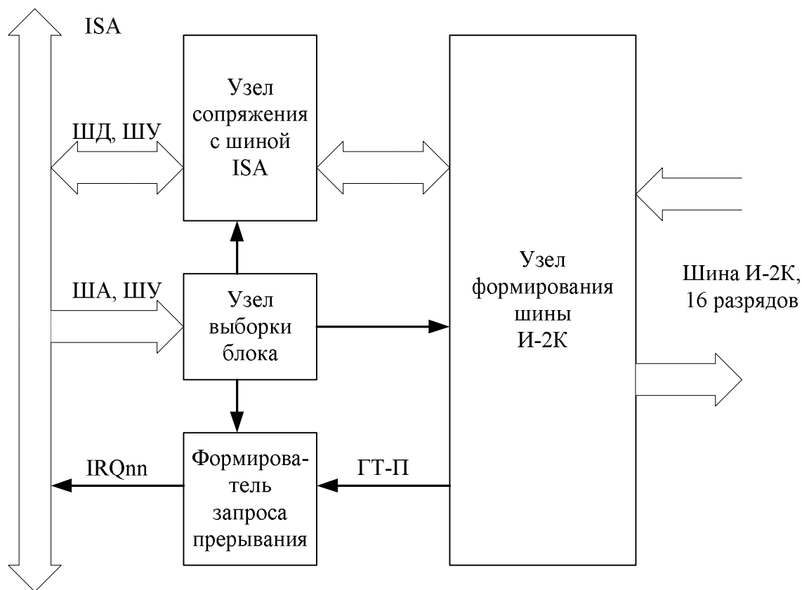
Рисунок 2 — Структура блока сопряжения РС с интерфейсом И-2К
