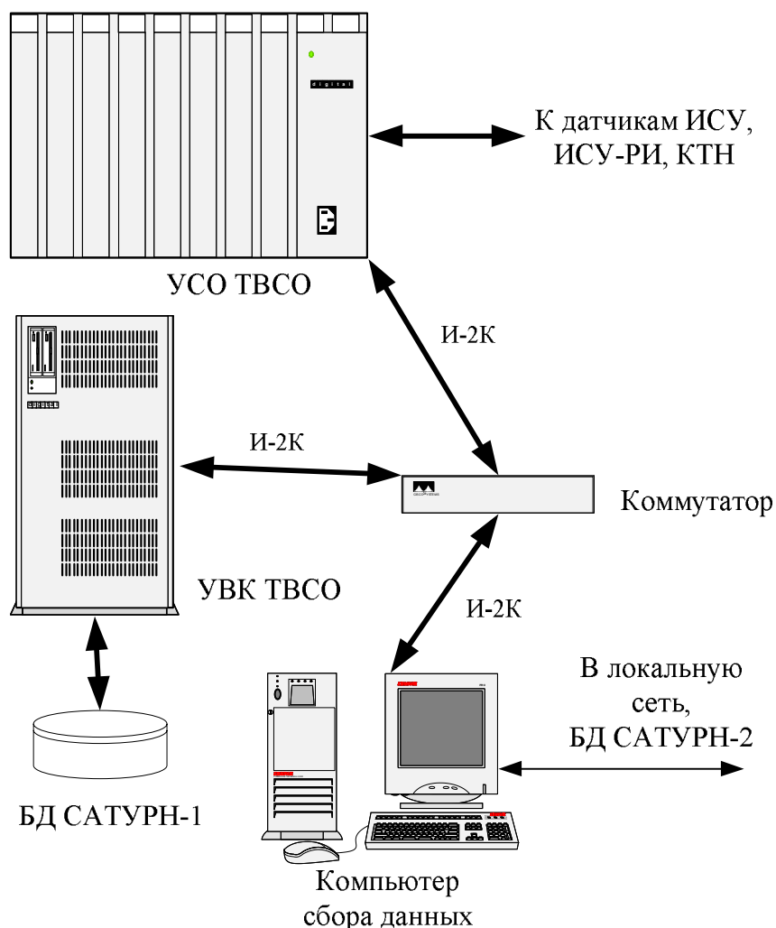
Рисунок 1 — Структурная схема системы сбора данных
