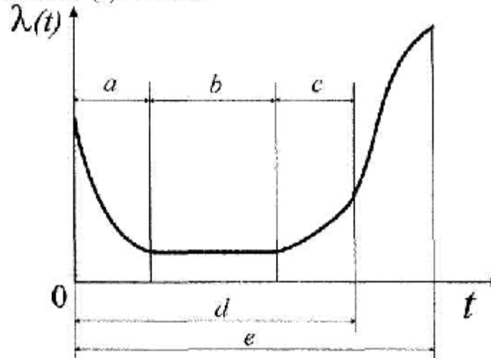
Рис. 2. Классическая кривая отказов (кривая «ванна»)
