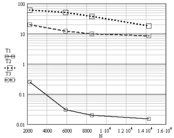
Рисунок 9 – Залежність швидкості реконструкції та візуалізації (fps) від кількості точок об'єкту для різних варіантів апаратної реалізації
