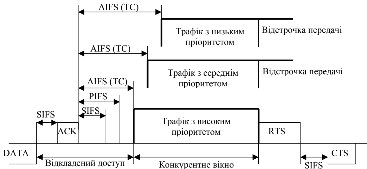
Рисунок 1 — Схема доступу трафіку з різним пріоритетом до середовища передачі
