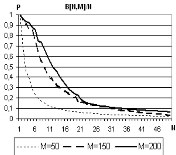
Рисунок 5 — Імовірність вдалої передачі бікону конкретним пристроєм в залежності від кількості пристроїв в мережі N при розмірі АТІМ-вікна M
