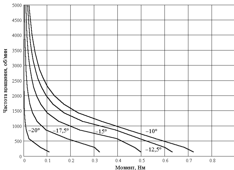
Рисунок 4 – Механические характеристики ВРД при широтно-фазовом управлении
