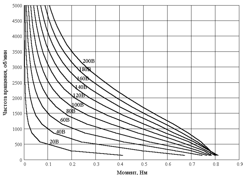
Рисунок 3 – Механические характеристики ВРД при управлении по уставке напряжения
