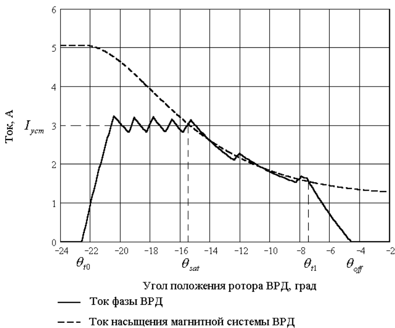
Рисунок 1 – Управляющие параметры ВРД
