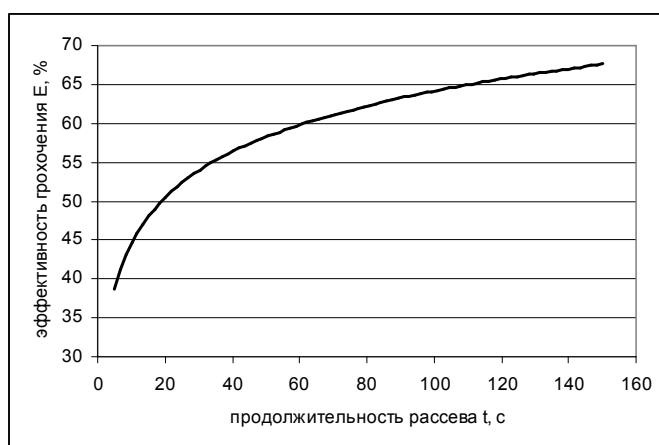
Рис. 1. Кинетика грохочения отходов строительных материалов
