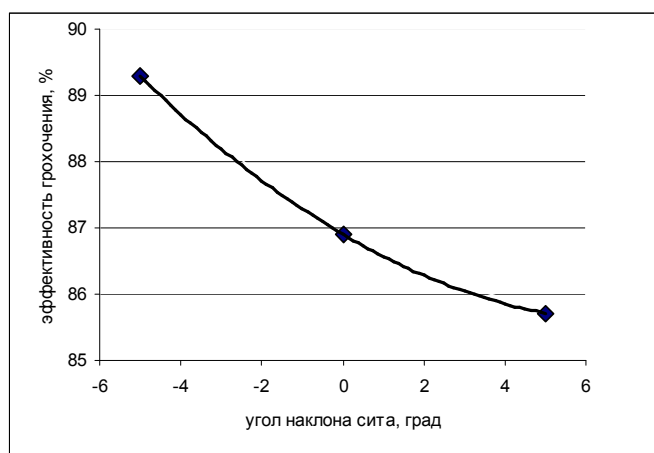
Рис. 2. Экспериментальная зависимость эффективности грохочения строительных отходов от угла наклона сита
