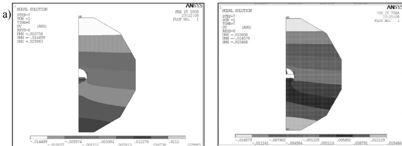
Рис. 4. Распределение вертикальных смещений в модели: а– без отпора по почве выработки, б– с отпором 3 кПа
