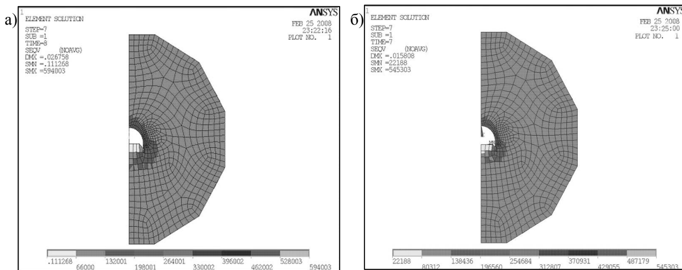
Рис. 3. Картина распределения в модели эквивалентных напряжений, рассчитанных по энергетической теории: а– без отпора по почве выработки, б– с отпором 3 кПа
