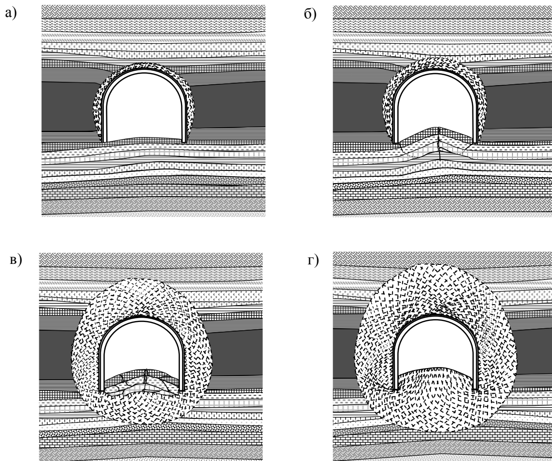
Рис. 1. Схемы механизма пучения почвы выработки на разных этапах ее существования: а, б- складкообразование породных слоев за счет формирования зоны разрушения вокруг выработки; в- выдавливание разрушенных пород в полость выработки под действием веса вышележащих пород, вмещающих ЗРП; г- выдавливание пород почвы вследствие нарушения равновесного состояния системы «крепь- ЗРП- окружающий породный массив»
