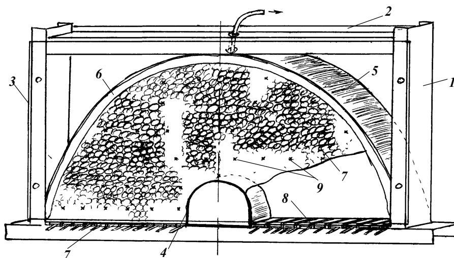
Рис. 2. Общий вид модели
