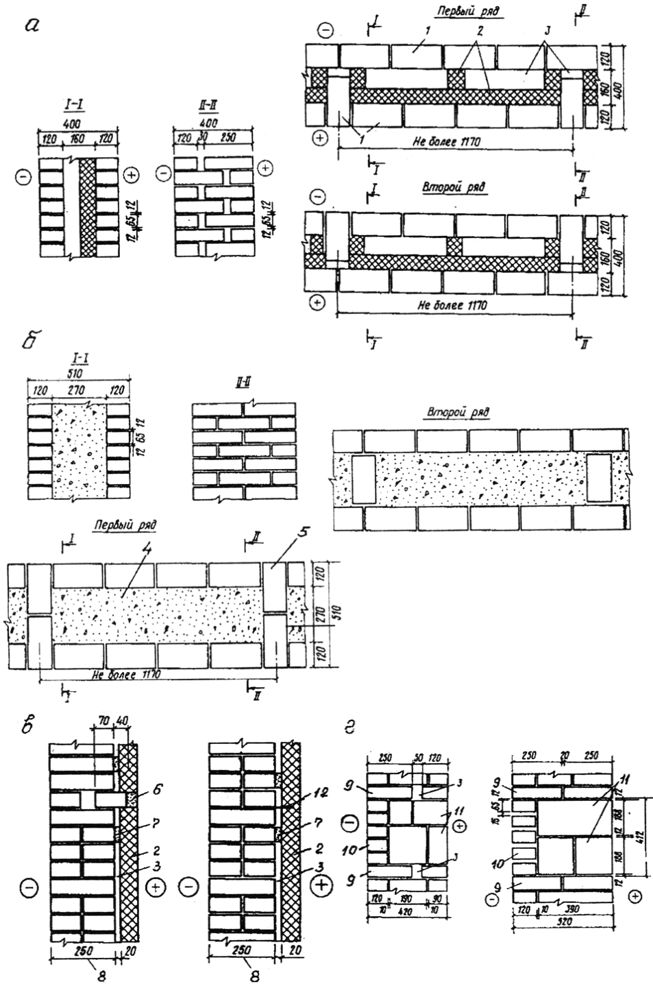
Рис. 1.14. Типы стен облегченной кладки:
