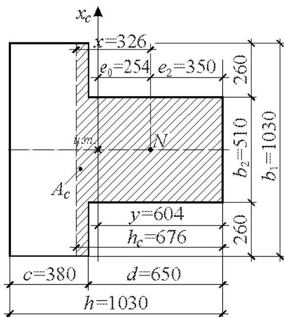
Рис. 5.3. Тавровое сечение
