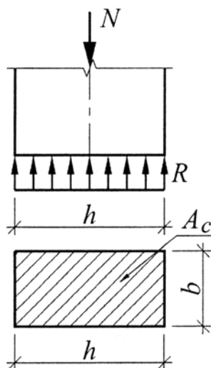
Рис. 3.2. К расчету каменной кладки при центрально сжатии
