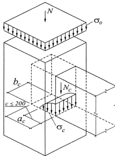
Рис. 3.6. Схема нагружения кладки местной и основной нагрузками
