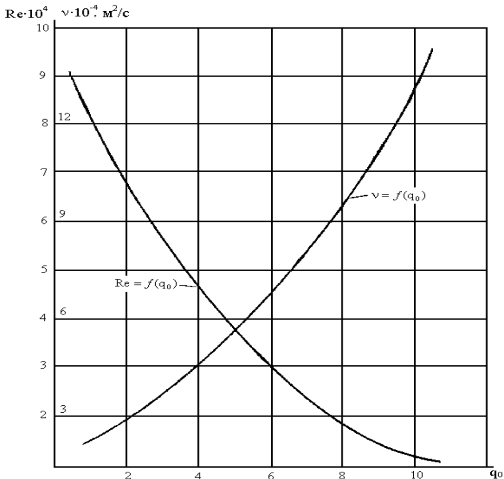
Рис. 4. Зависимость числа Рейнольдса и кинематической вязкости от относительного расхода воздуха
