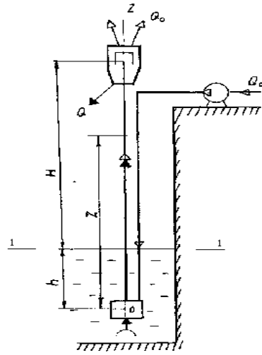
Рис.2. Расчетная схема эрлифта
