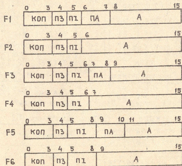
Рис. 2. Форматы команд
