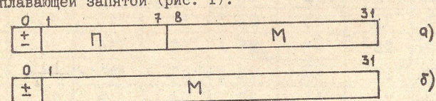
Рис. 1. Формат операндов:
