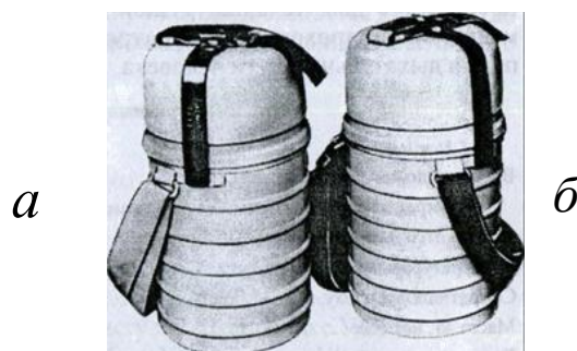
Рис. 4.1 – Шахтный изолирующий самоспасатель ШСС-1 в двух исполнениях: а) корпус из углеродистой стали; б) из нержавеющей стали
