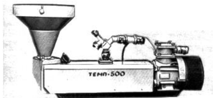
Рис. 8.1 – Комплекс для дистанционного возведения безрубовых перемычек «Темп-500»
