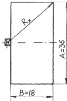
Рис.9.1 План расположения здания и молниеотвода
