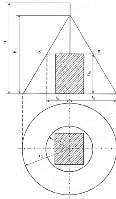
Рис. 9.2 Зона защиты молниеотвода
