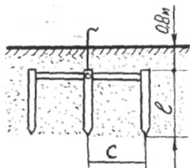
рис.9.3 Заземли- тель молниеот- вода
