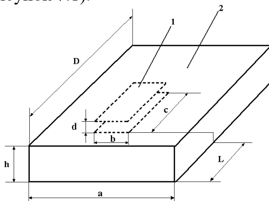
Рисунок 7.1. Конденсатор установки диэлектрического нагрева (1) с прямоугольным трубчатым экраном (2).
