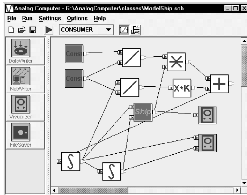
Рис. 2 - Фрагмент схеми моделювання динаміки судна
