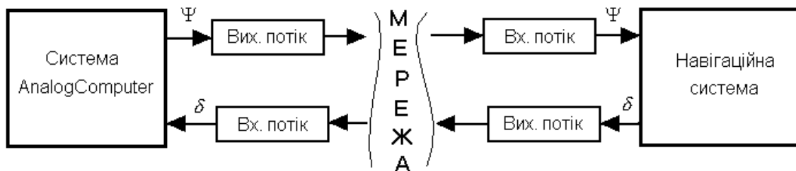
Рис. 3 - Структура розподіленого моделювання
