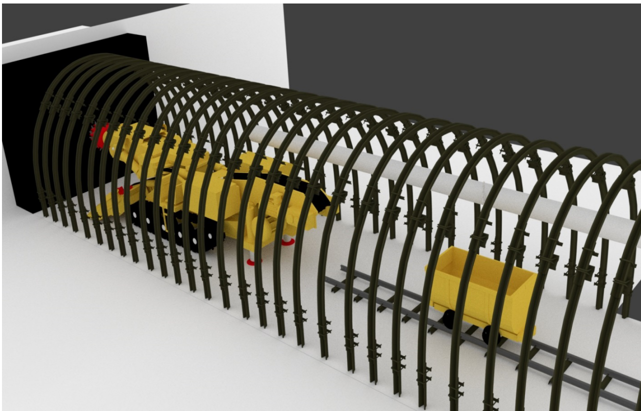
Рисунок 2 – Модель проходческих работ
