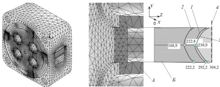
Рисунок 5. Конечно-элементная модель A и эпюры эквивалентных напряжений B : 1 – температура 300 °С; 2 – температура 250 °С; 3 – совместное действие температуры 300 °С и давления в цилиндре 2,1 МПа; 4 – предел текучести чугуна ВЧ50 \sigma_{0,2} = 320 МПа
