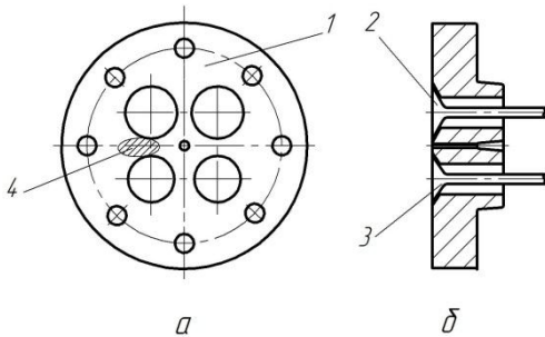
Рисунок 3. Схема огневого днища крышки цилиндра: а – вид со стороны рабочих газов; б – разрез по клапанному отверстию; 1 – крышка цилиндра; 2 – впускной клапан; 3 – выпускной клапан; 4 – трещины
