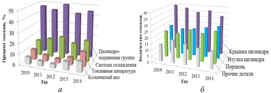
Рисунок 1. Распределение неисправностей узлов силовой дизельной установки горно-транспортной машины: а – всего двигателя; б – деталей цилиндрической группы
