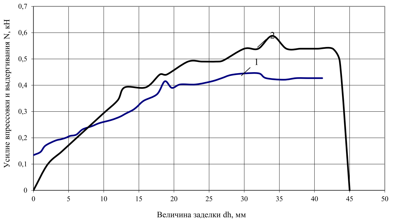
Рис. 1 – Зависимость усилия впредования и выдергивания анкера с распорной втулкой от величины заделки
