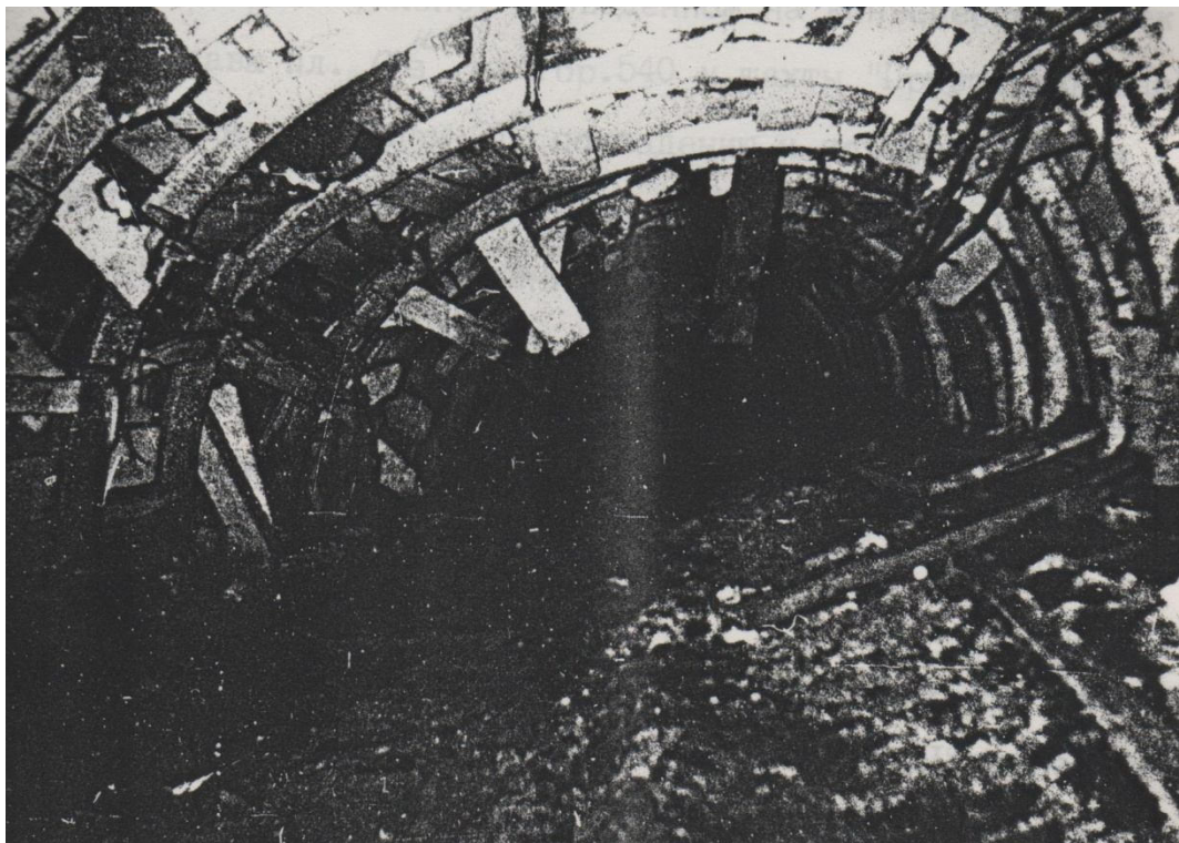
Рис. 1. Проявление неравномерности смещений пород по контуру выработок: а – в 8-м западном полевом штреке гор. 840м шахты «Новодружеская»; б – в 7-м западном полевом вентиляционном штреке пласта \sigma_{33} гор. 650м шахты им. Г.Г. Капустина
