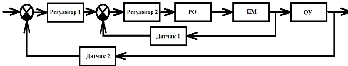
Рисунок 4 – Двухконтурная система управления
