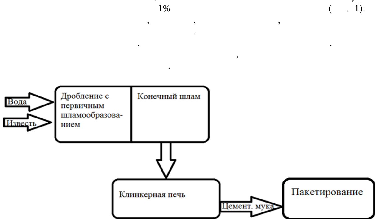
Рисунок 1 – Схема производства цементной муки
