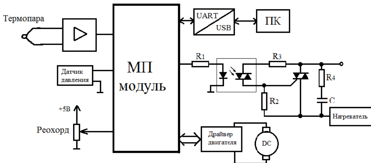
Рисунок 3 – Предложенная структурная схема разрабатываемой электронной системы
