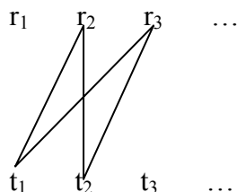
Рис. 1. Граф.
