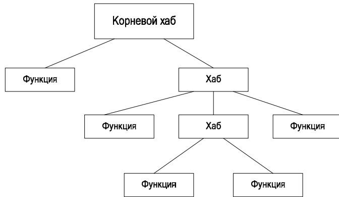
Рисунок 1 – Физическая топология шины USB
