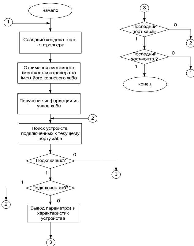
Рисунок 3 – Алгоритм идентификации USB-
