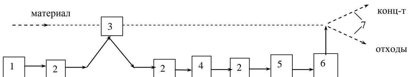
Рис 2.3. Схема сортировки полезных ископаемых:
