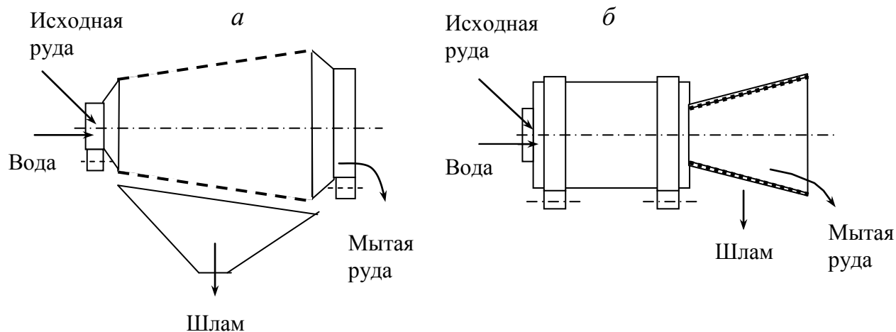
Рис. 11.3. Схемы бутары (а) и скруббер-бутары (б)
