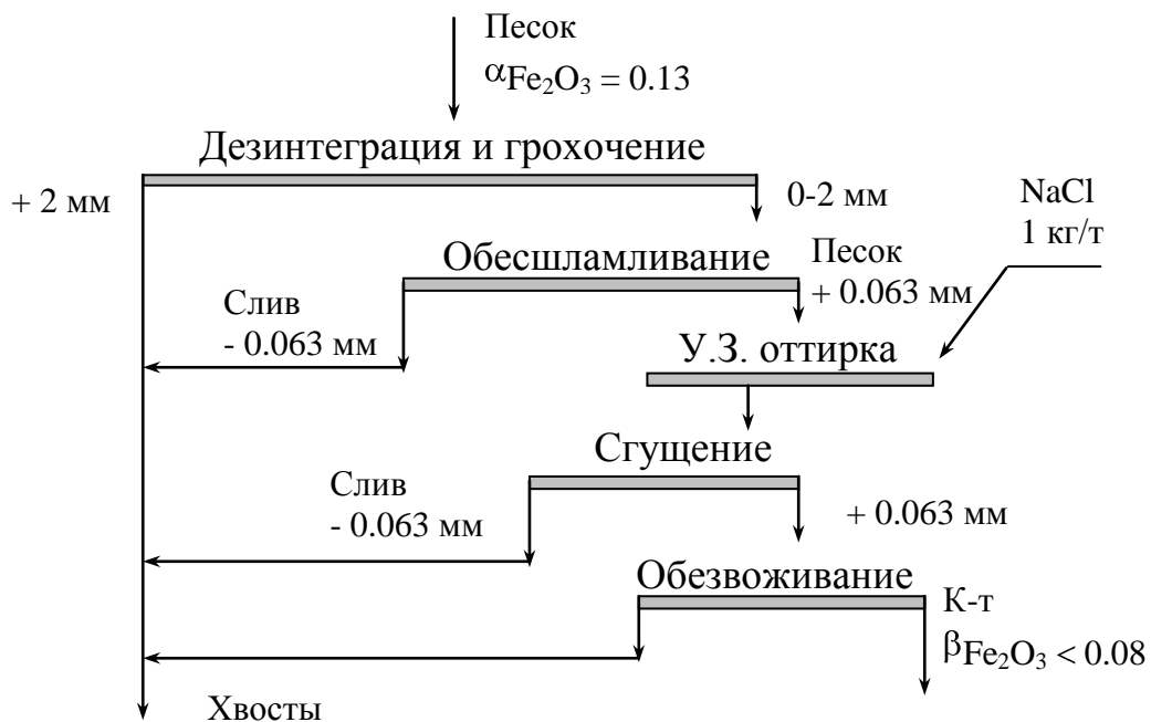
Рис. 12.7. Схема обогащения кварцевого песка
