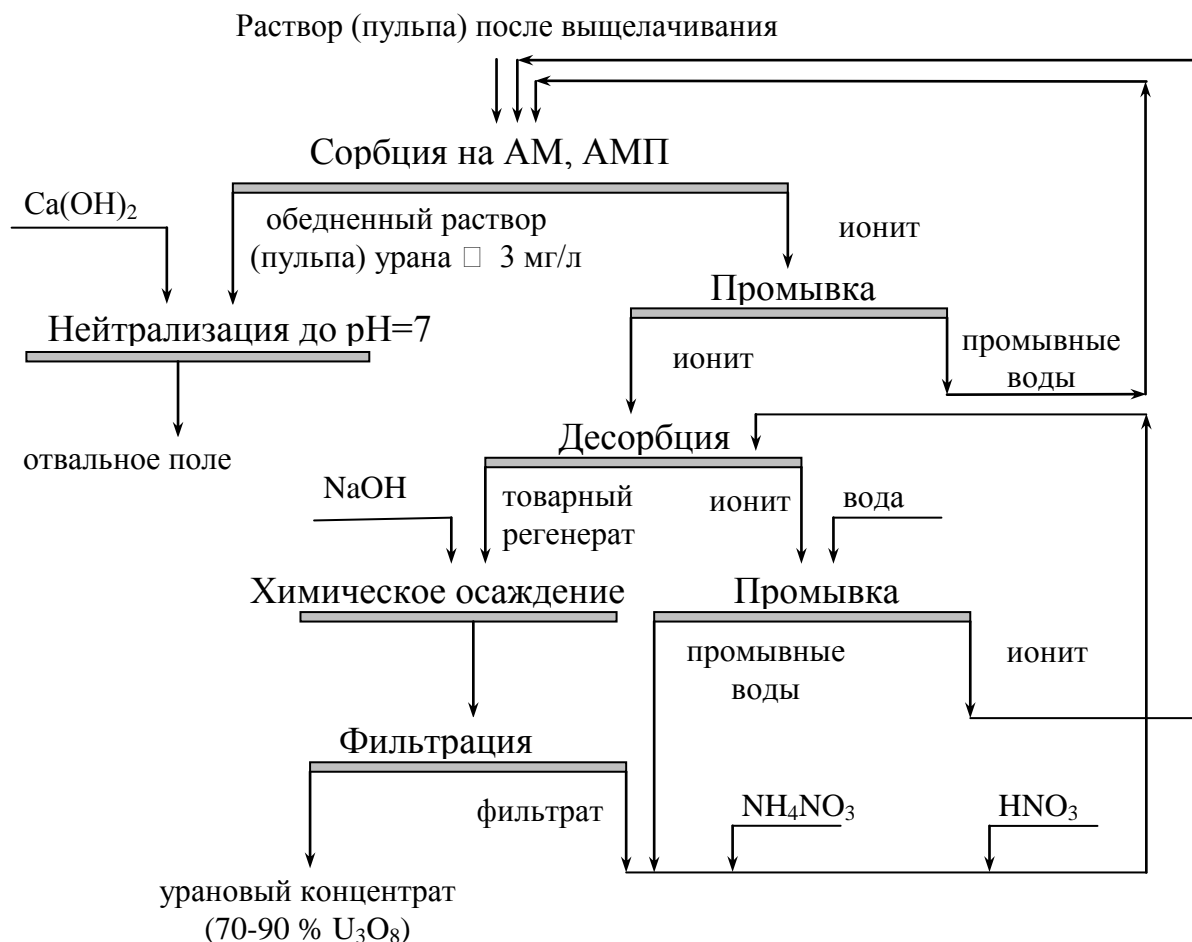
Рис. 22.2. Технологическая схема анионообменного извлечения урана из серноокислых растворов (пульпы)
