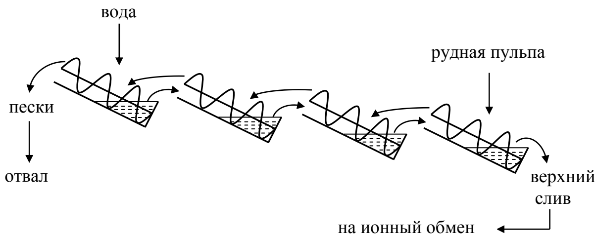
Рис.22.1. Схема противоточной отмывки песков
