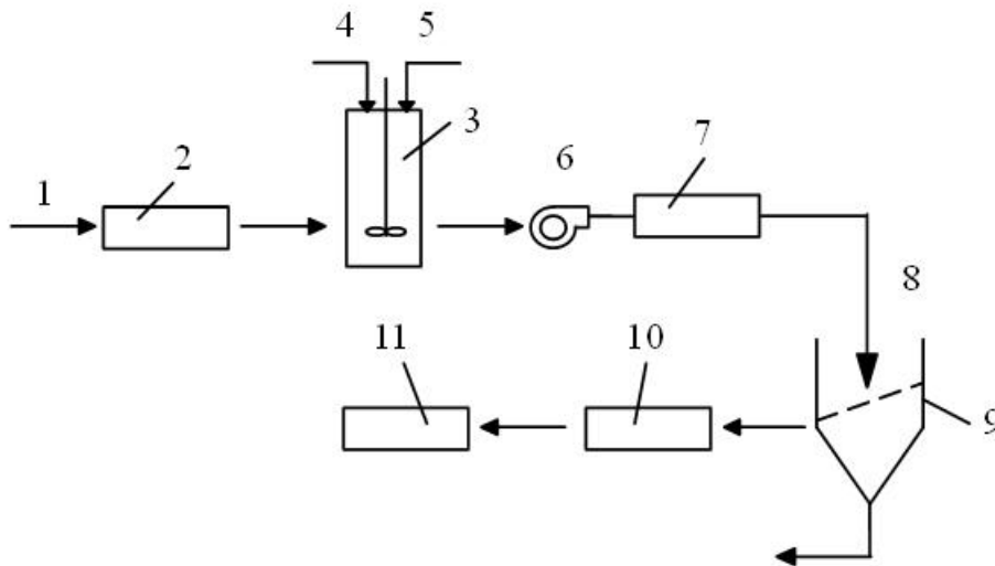
Рис. 15.2 – Схема масляной агрегации с использованием углепровода, как гранулятора:
