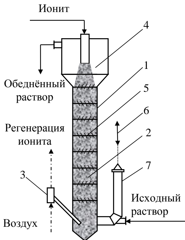
Рис. 18.3. Колонна ПСК-Р:
