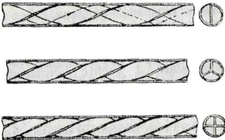
Рис. 15.3. Разрезы трубопровода-гранулятора
