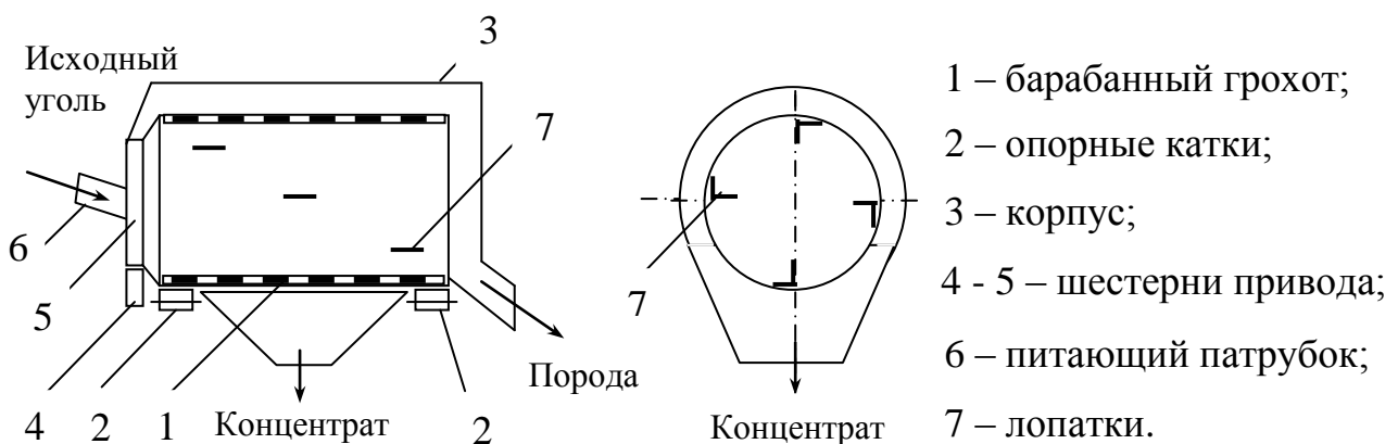
Рис. 10.2. Дробилка полужесткого дробления
