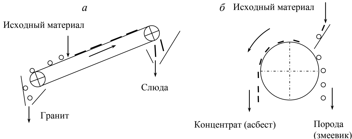
Рис. 8.6. Сепараторы трения: а - ленточный; б – барабанный
