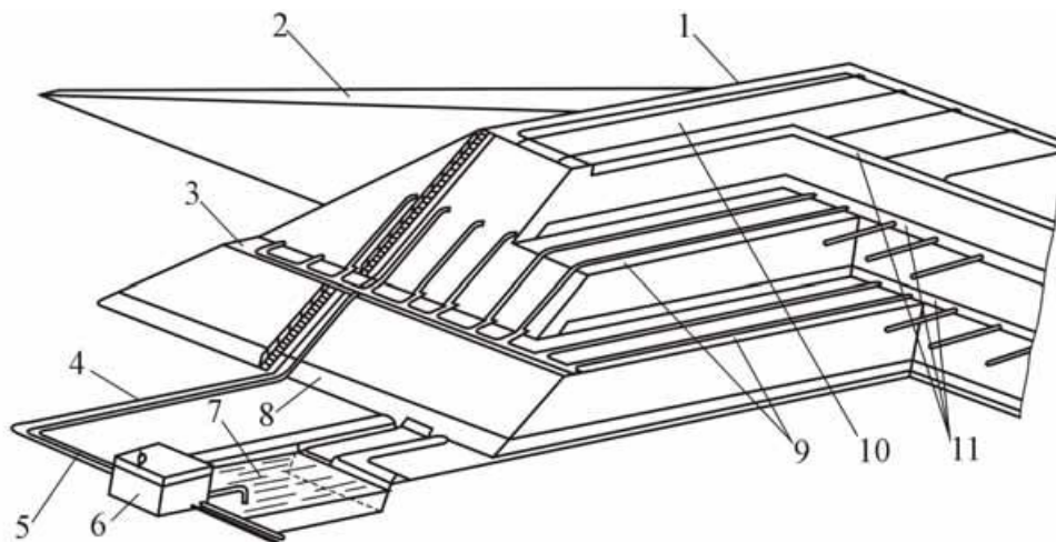
Рис. 17.5. Кучное выщелачивание:
