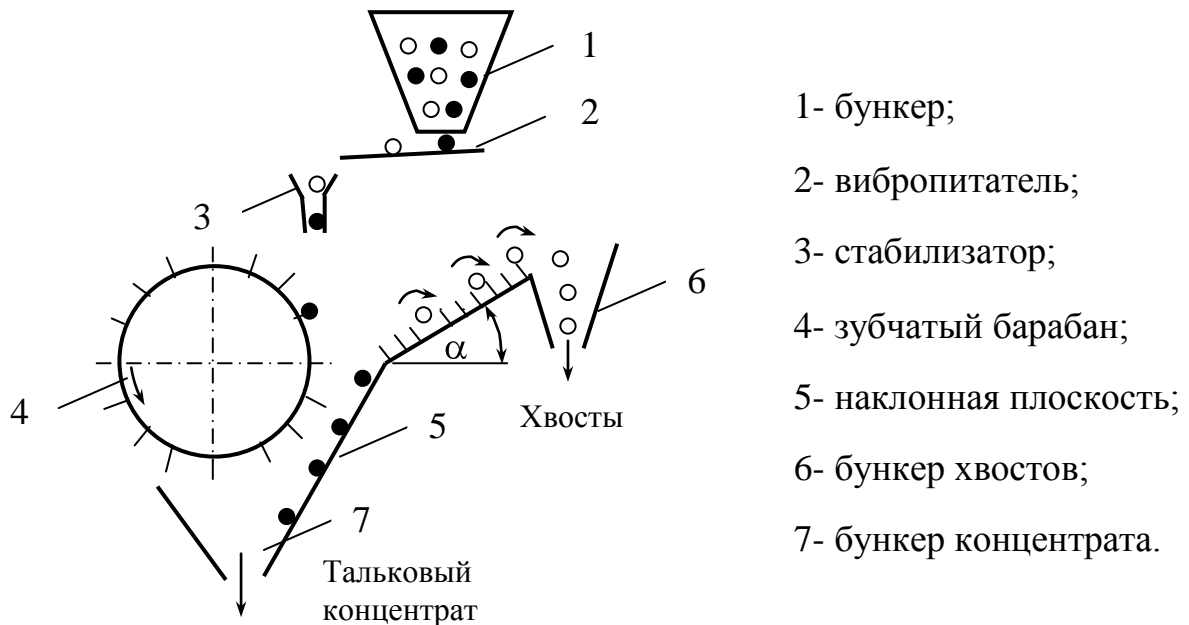
Рис. 8.8. Схема сепаратора ВНИИНеруд
