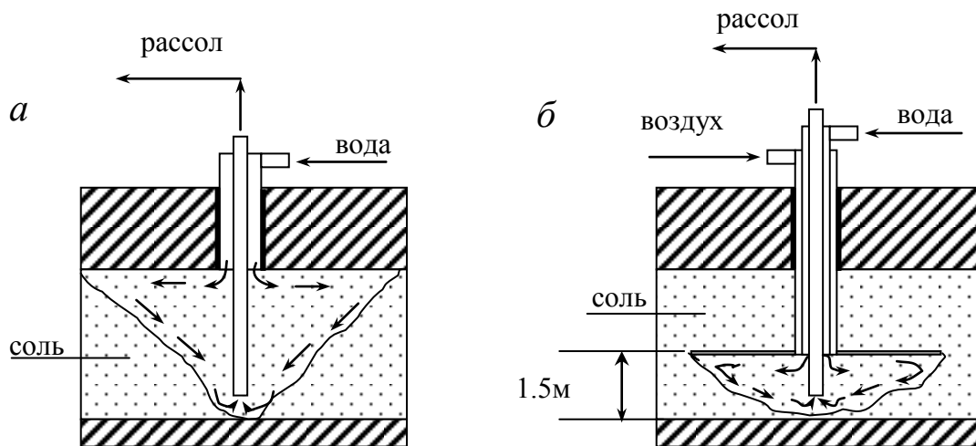
Рис.19.3. Схема выщелачивания пласта соли через буровую рассольную скважину: а – противоток, б - гидровруб
