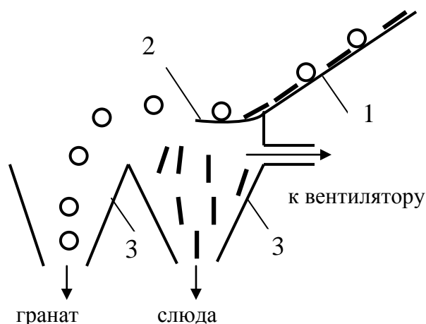
Рис. 9.3. Полочный сепаратор
