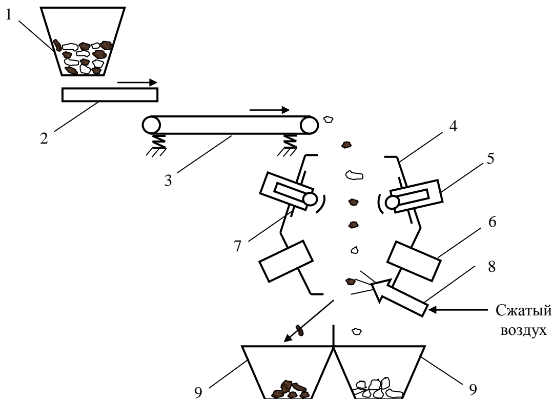
Рис. 6.1. Схема фотометрического сепаратора:
