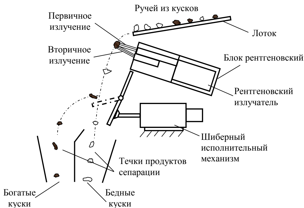
Рис. 7.1. Схема работы сепаратора СРФ
