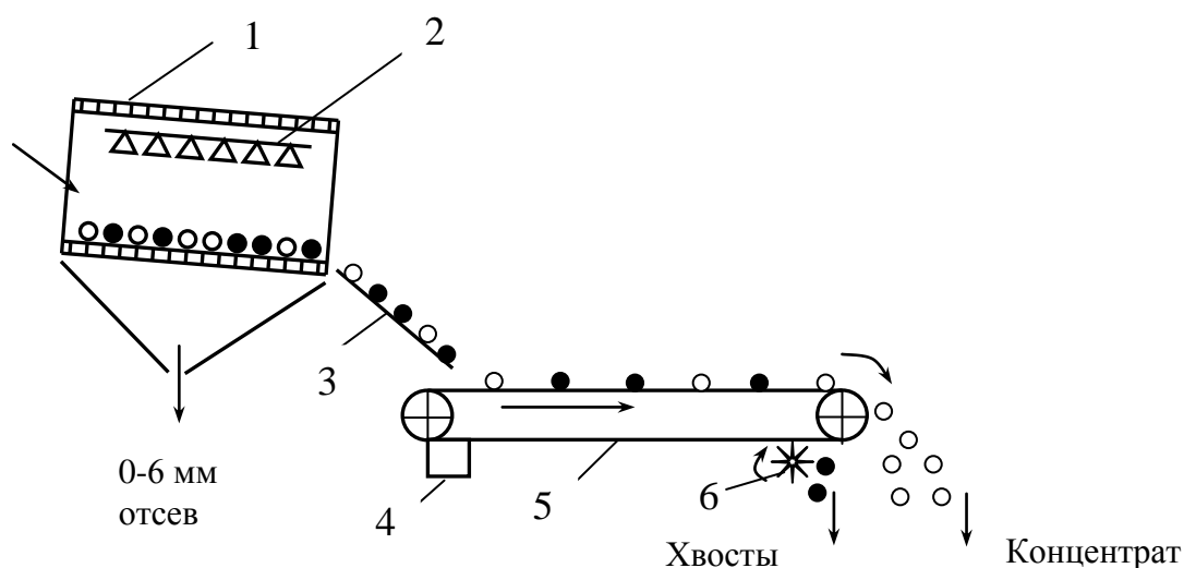
Рис. 9.6. Схема термоадгезионного сепаратора
