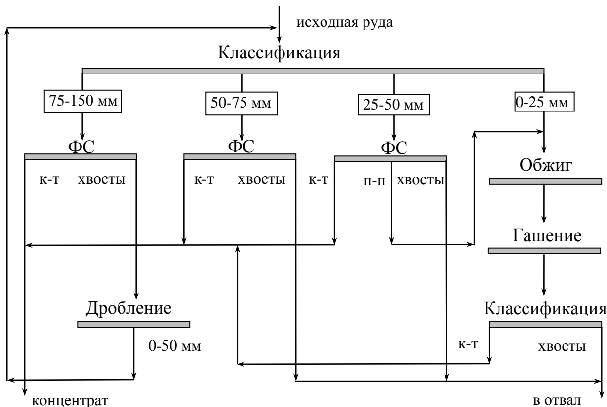
Рис. 6.3. Схема обогащения фосфоритов Обладжанского месторождения
