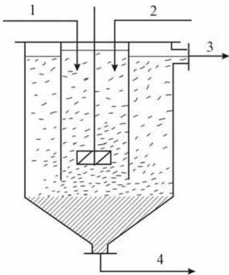
Рис. 18.8. Схема внутреннего смесителя-отстойника: 1 – исходный раствор; 2 – экстрагент; 3 – экстракт; 4 – рафинат.
