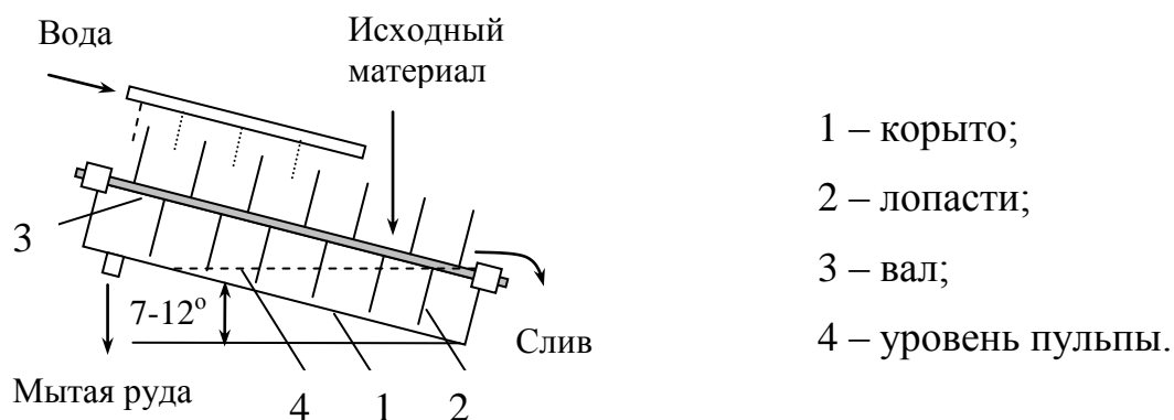
Рис. 12.2. Наклонная корытная мойка
