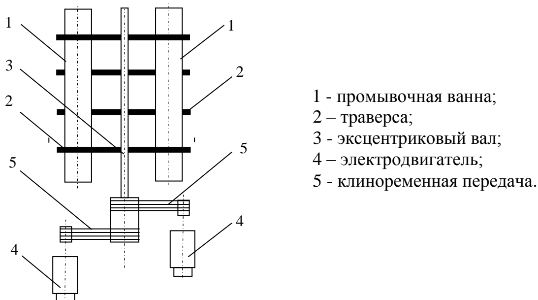
Рис. 12.3. Схема вибромойки СМД-88
