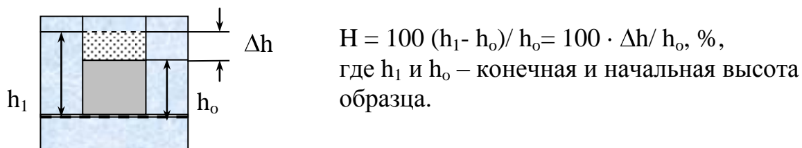
Рис. 11.2. Схема набухания глины
