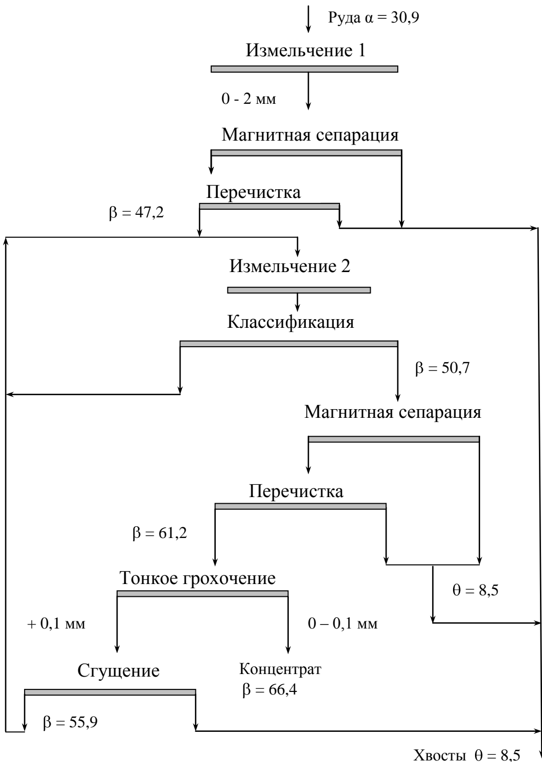
Рис. 10.4. Схема переработки магнетитовых руд
