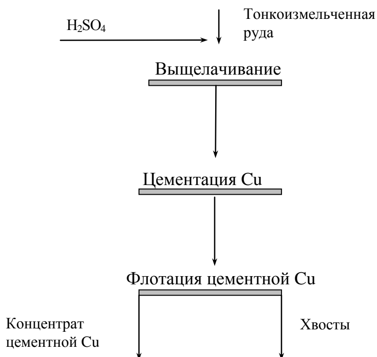
Рис. 19.4. Принципиальная схема переработки труднообогатимых медных руд по методу Мостовича
