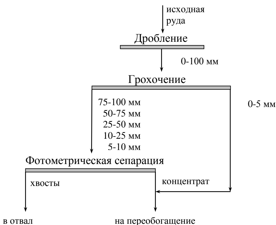
Рис. 6.2. Схема фотометрической сепарации золотосодержащих руд
