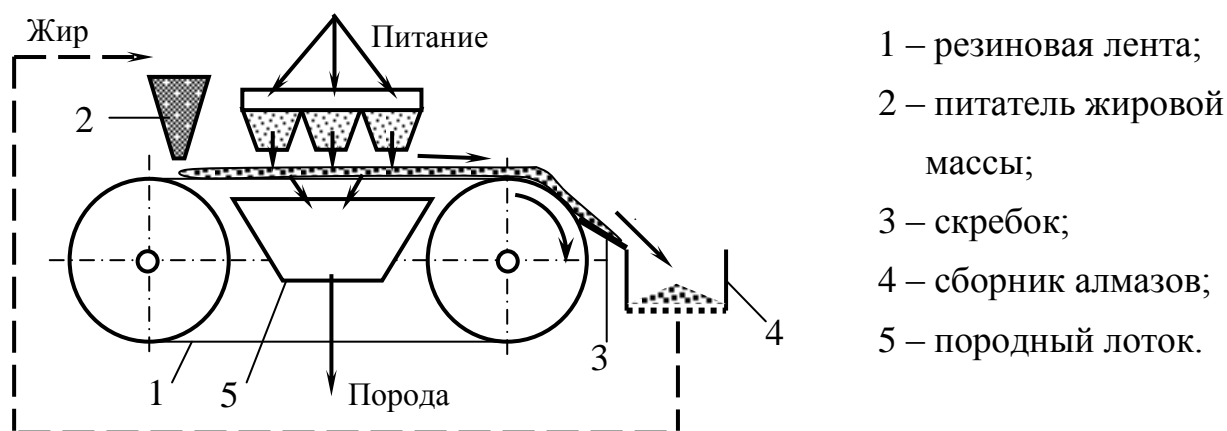
Рис. 9.7. Ленточный жировой стол
