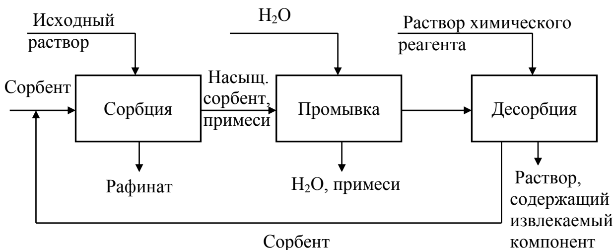
Рис. 18.2. Общая схема концентрирования металлов
