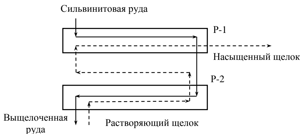
Рис. 19.2. Схема движения руды и растворителя в шнековых растворителях (P-1 и P-2) при противоточном методе растворения
