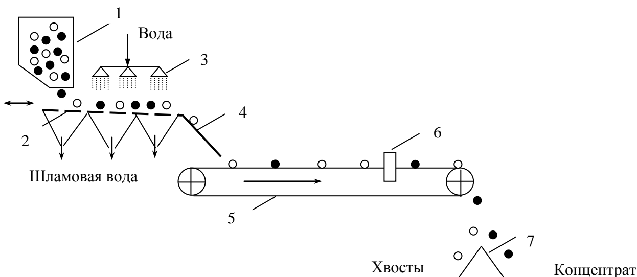
Рис. 3.5. Статистическое формирование покусковой подачи с промывкой материала:
