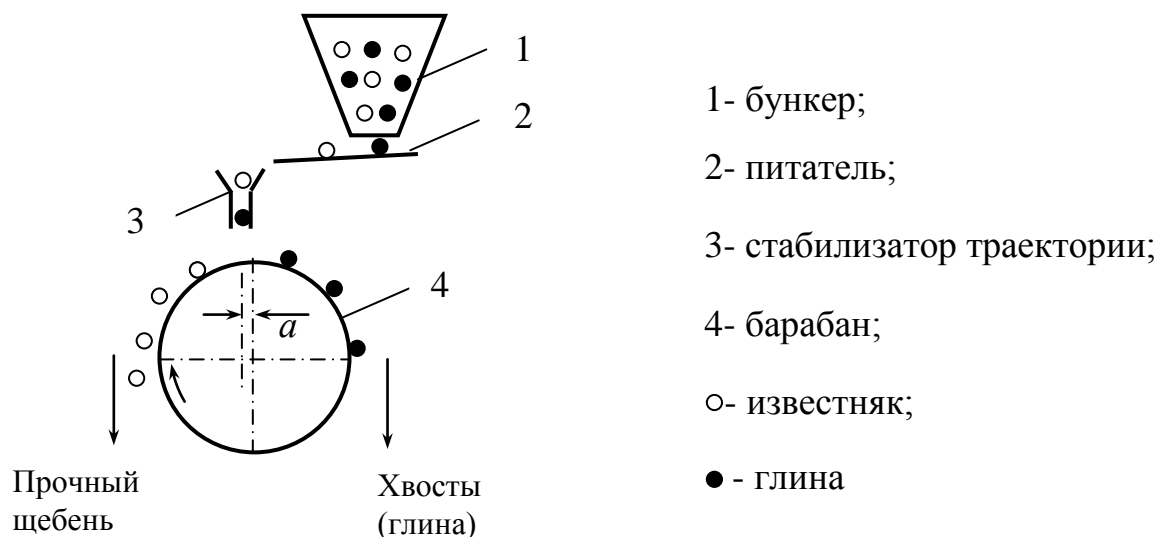
Рис. 8.7. Схема однобарабанного сепаратора Н.К. Тимченко
