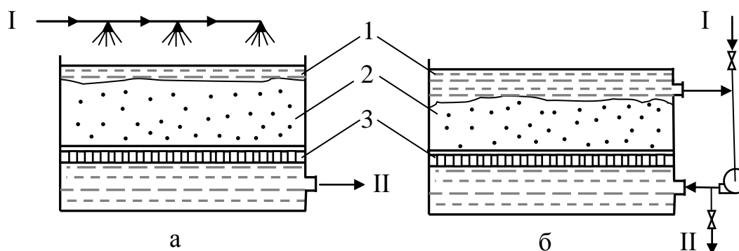
Рис. 17.4. Аппараты (перколяторы) для перколяционного выщелачивания: а – с движением раствора под действием силы тяжести (сверху вниз); б – с принудительной циркуляцией раствора (снизу вверх); I – выщелачивающий раствор, II – раствор на дальнейшую переработку; 1 – корпус; 2 – выщелачиваемый материал; 3 – дренажное устройство; 4 – насос
