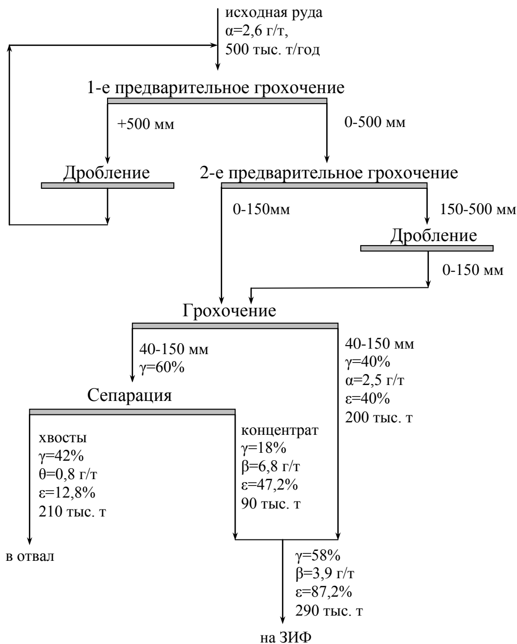
Рис. 7.3. Технологическая схема предварительного обогащения золотосодержащих руд месторождения Эльдорадо
