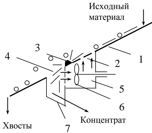
Рис. 9.4. Плоскостной сепаратор
