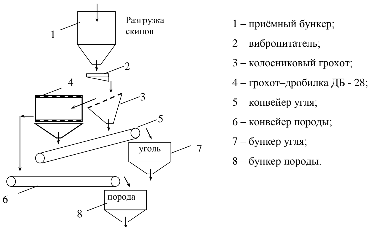
Рис. 10.3. Схема установки избирательного дробления
