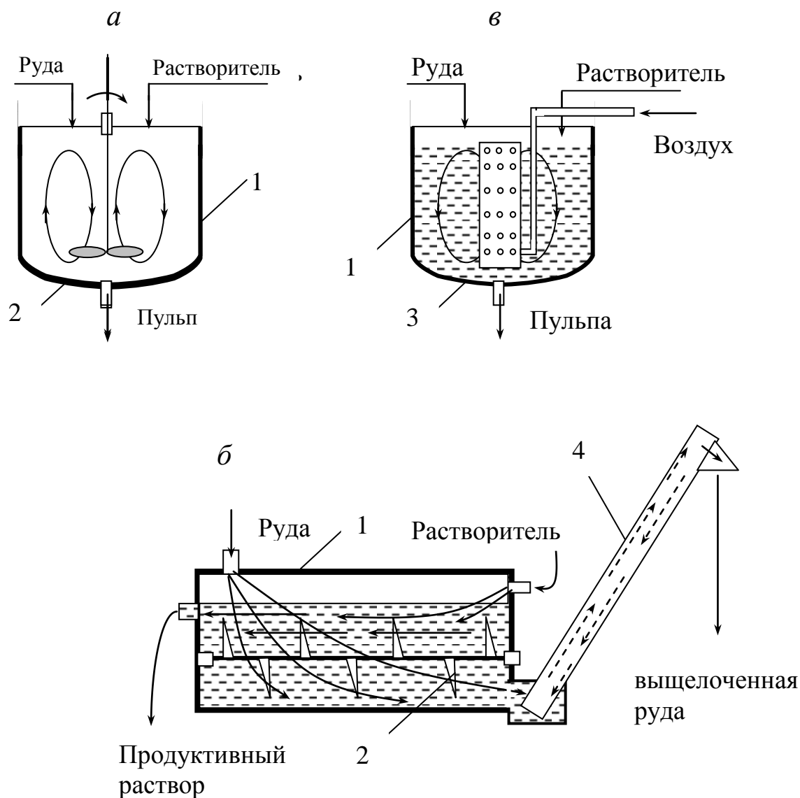
Рис. 17.1. Схема чанов с перемешивающим устройством вертикального (а), горизонтального типа (б), пневматического (в) типов:
