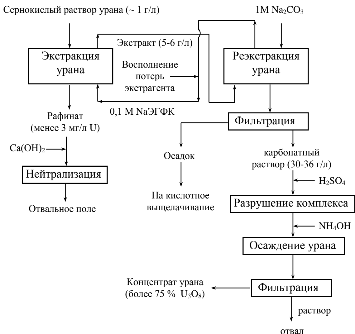
Рис. 22.3. Технологическая схема экстракции урана растворами ЭГФК
