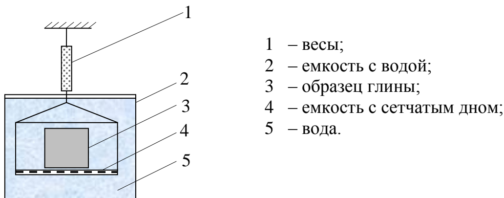
Рис. 11.1. Определение размокаемости глины
