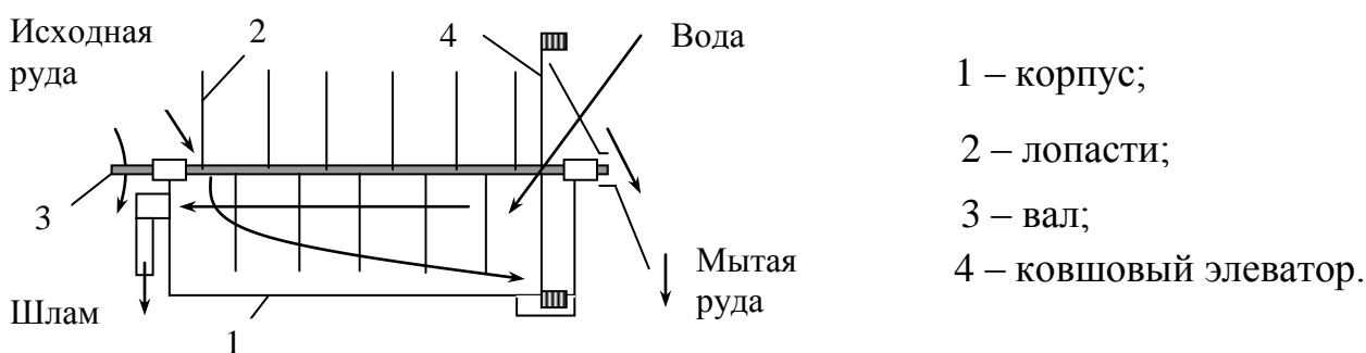
Рис. 12.1. Горизонтальная корытная мойка
