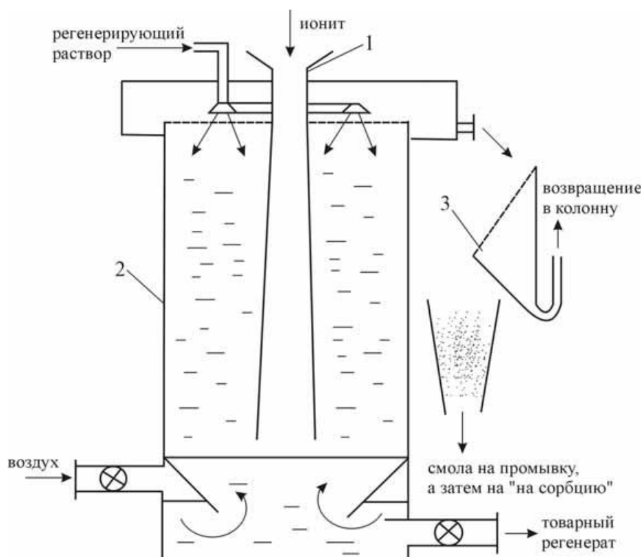
Рис. 18.5. Колонна КНСПР:
