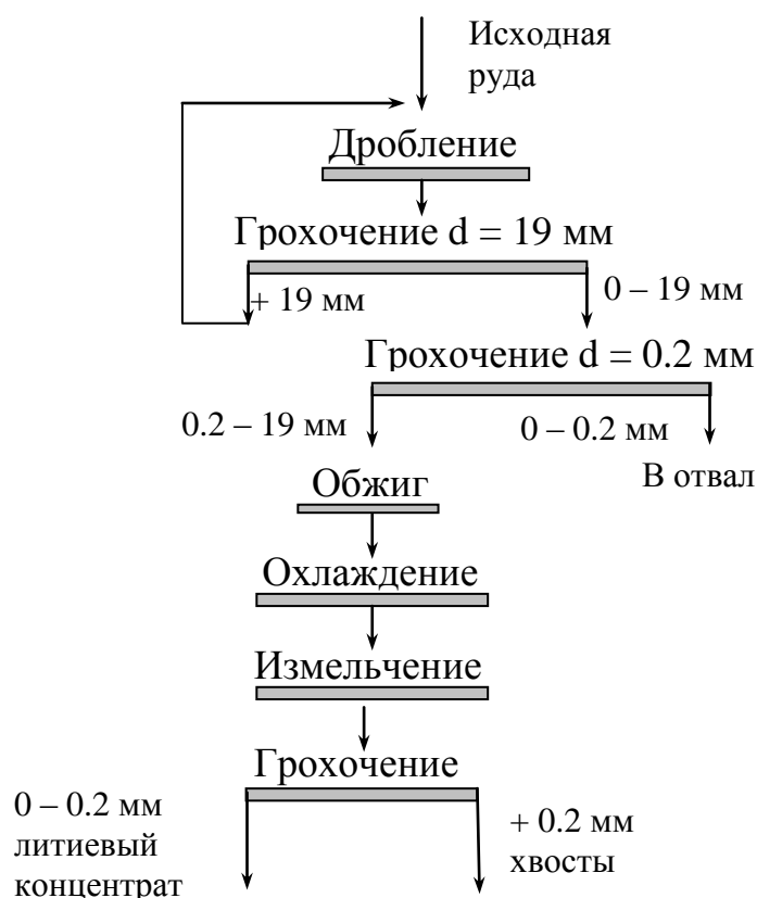
Рис. 13.1. Схема переработки сподуменовой руды
