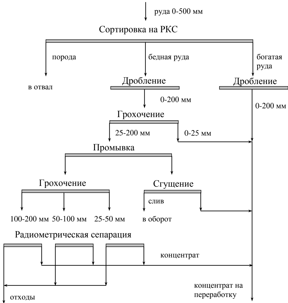
Рис. 4.2. Схема авторадиметрического обогащения урановой руды
