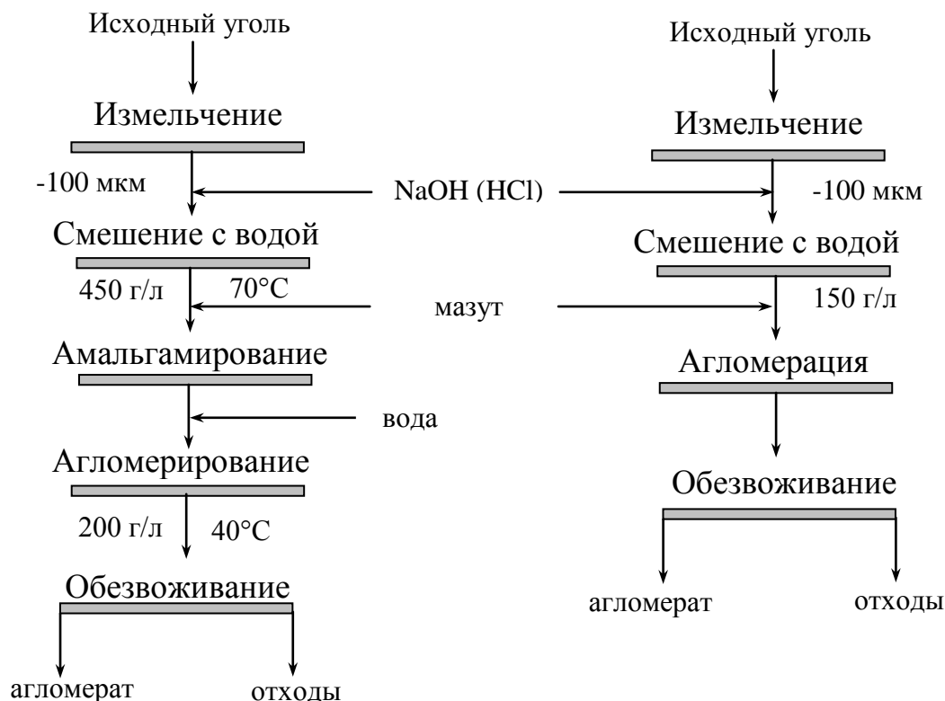
Рис. 15.1. Технологические схемы масляной агломерации в концентрированной (а) и разбавленной (б) суспензиях
