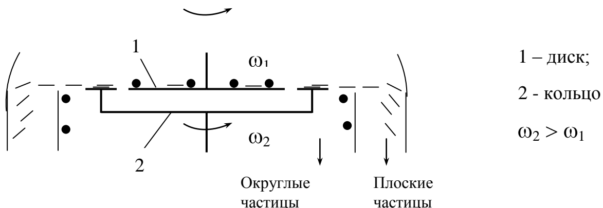
Рис. 9.5. Центробежный сепаратор
