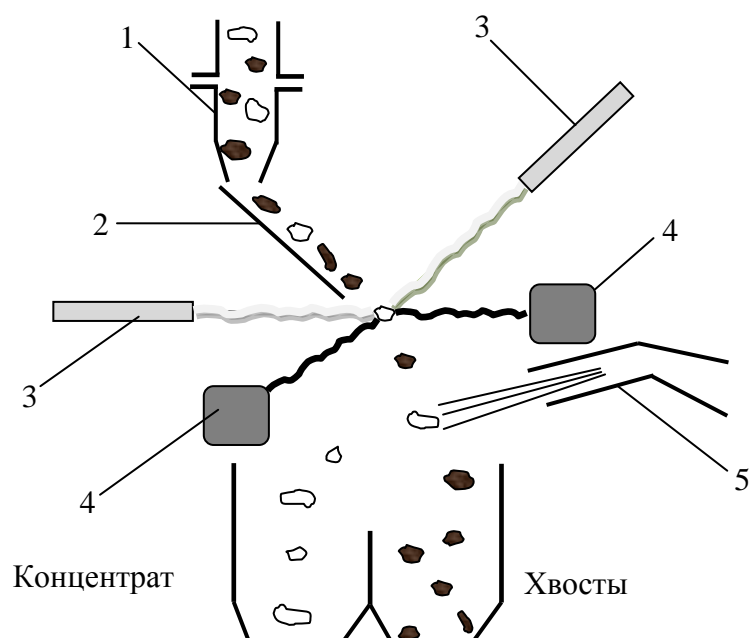
Рис. 5.1. Схема работы сепаратора ЛС-20-05Н:
