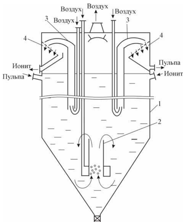
Рис. 18.4. Ионообменный пачук:
