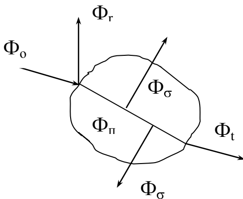
Рис. 2.1. Схема прохождения излучения через горную породу
