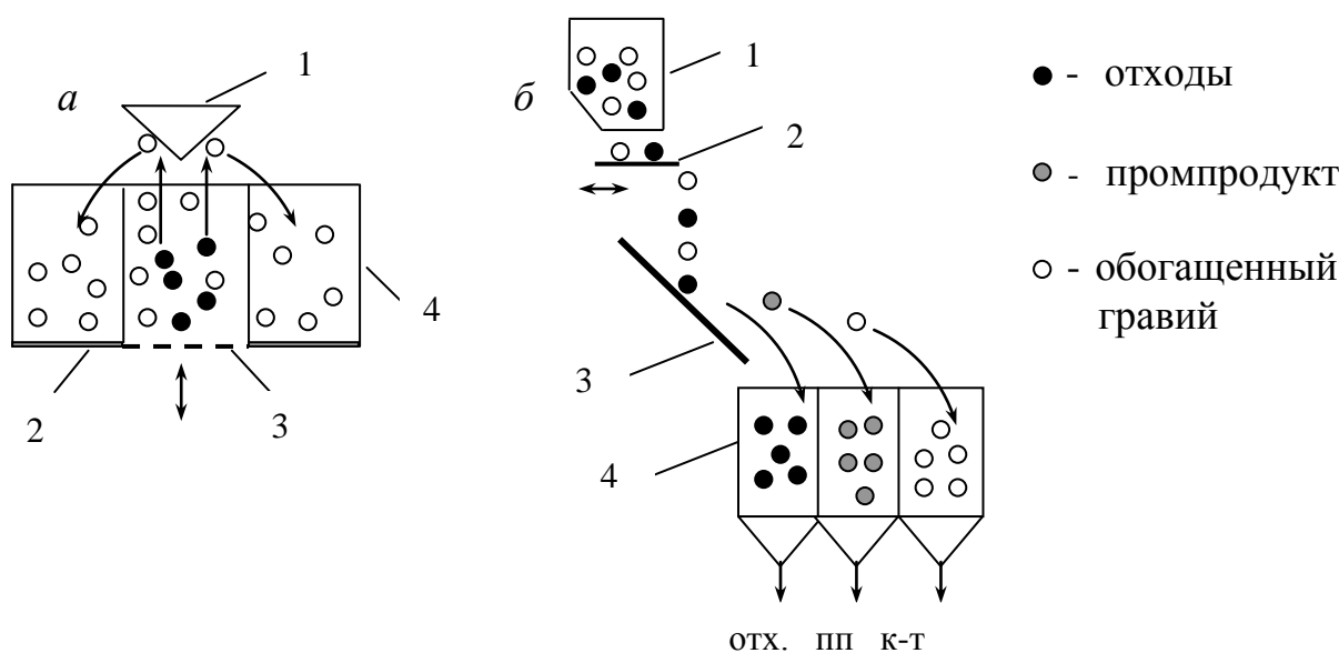
Рис. 8.2. Схемы сепараторов:
