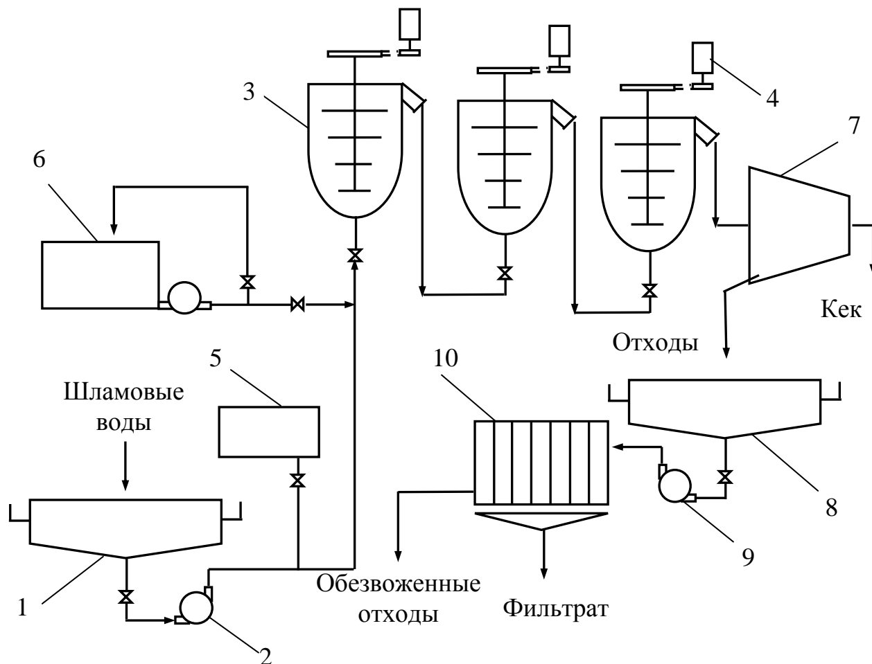
Рис. 14.1. Промышленная установка обогащения энергетических шламов селективной масляной флокуляцией на ЦОФ «Россия»:
