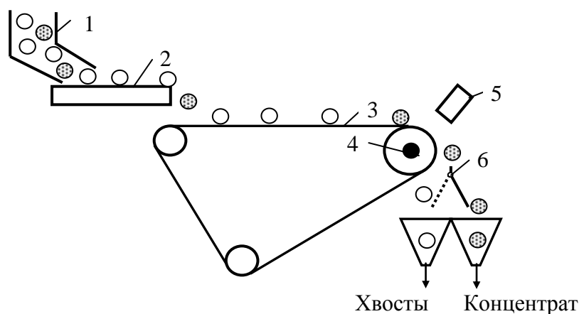
Рис. 6.4. Схема ленточного гамма-абсорбционного сепаратора РС-2Ж: 1 – бункер; 2 – вибропитатель; 3 – ленточный транспортёр; 4 – гамма-излучатель; 5 – датчик; 6 – шибер
