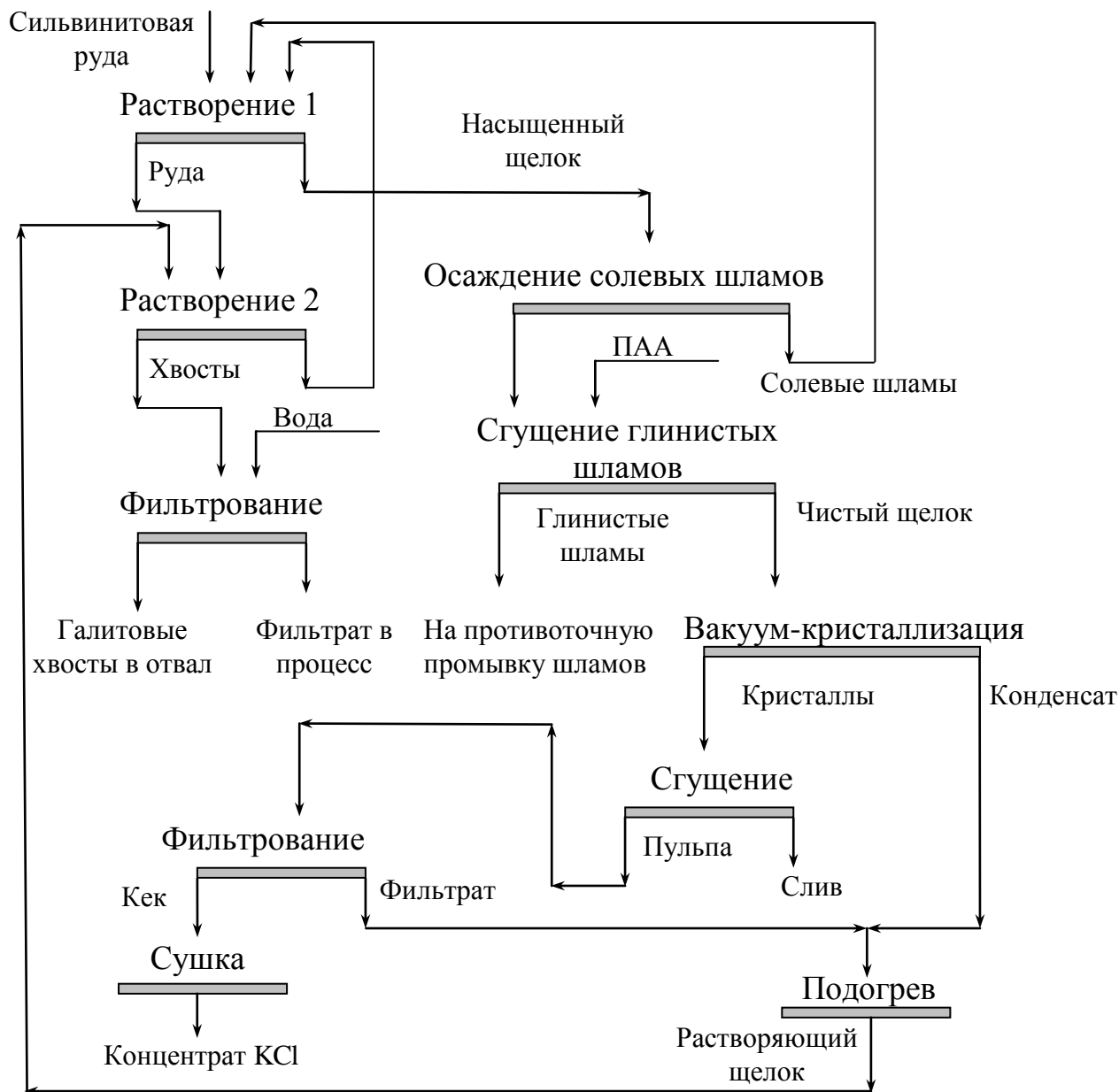
Рис. 19.1. Технологическая схема обогащения сильвинитовых руд
