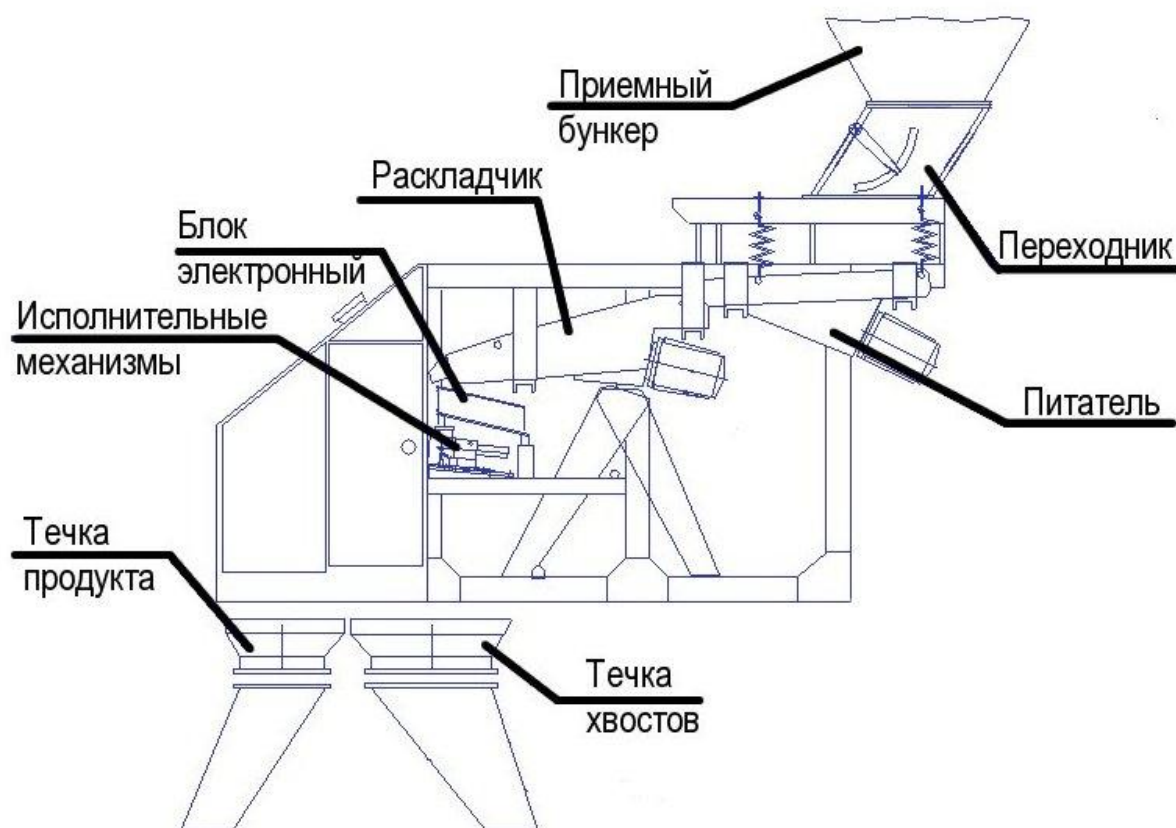
Рис. 7.2. Сепаратор СРФ-4-150
