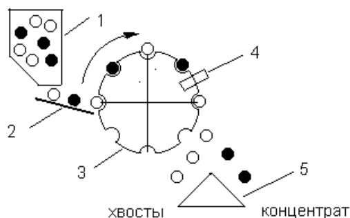
Рис 3.2. Детерминированное формирование покусковой подачи материала
