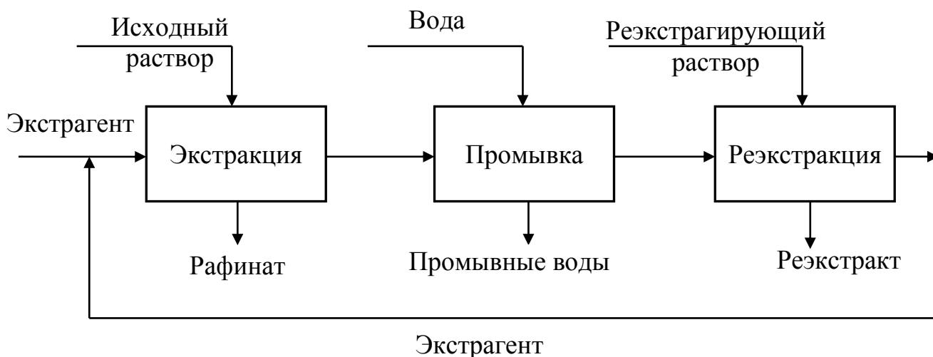
Рис. 18.6. Общая схема экстракционного концентрирования металлов
