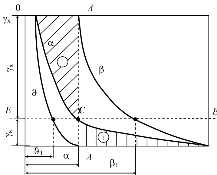
Рис. 2.4. Кривые обогатимости
