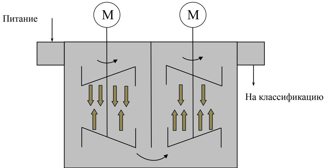
Рис. 12.6. Схема машины оттирочной МО-20
