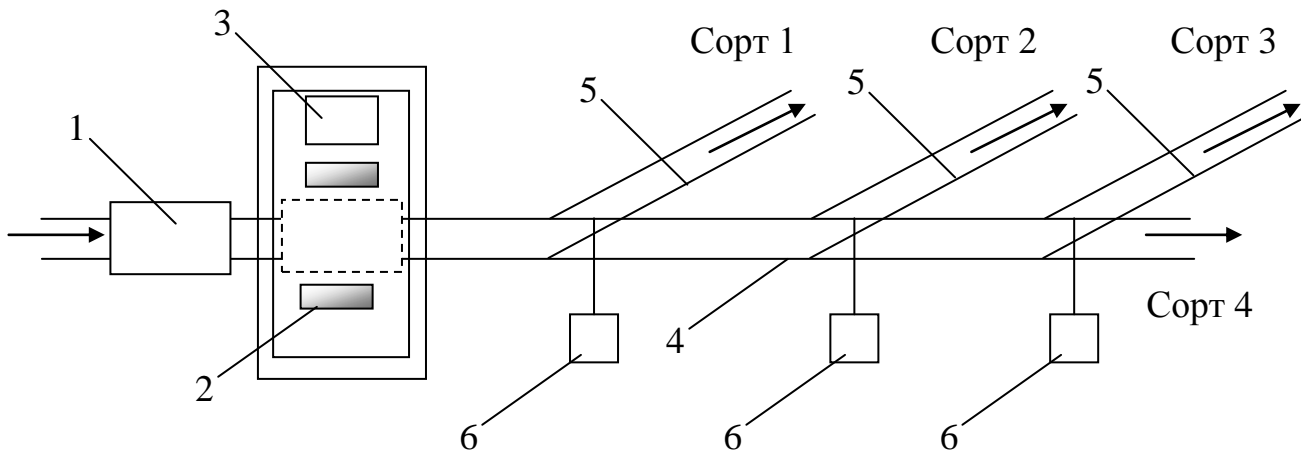
Рис. 3.1. Схема сортировочного пункта на РКС:
