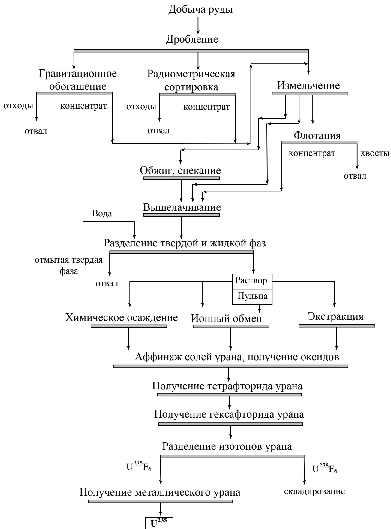
Рис. 21.1. Общая схема переработки урансодержащих руд
