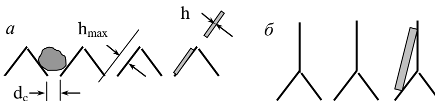
Рис. 9.1. Просеивающая поверхность: а- крышевидный грохот; б- крышевидный грохот с вертикальными перегородками
