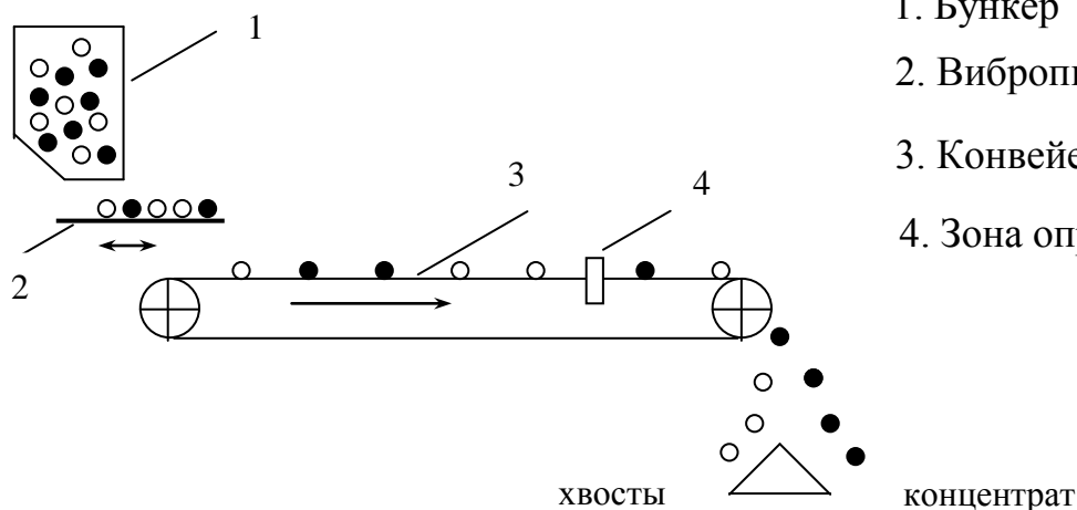
Рис. 3.3. Статистическое формирование покусковой подачи материала
