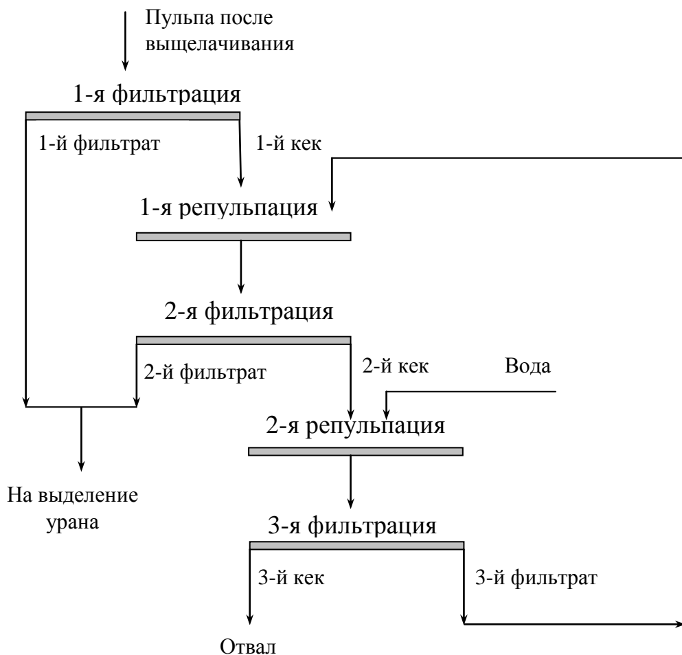
Рис. 18.1. Общая схема проведения процесса отмывки осадка после выщелачивания
