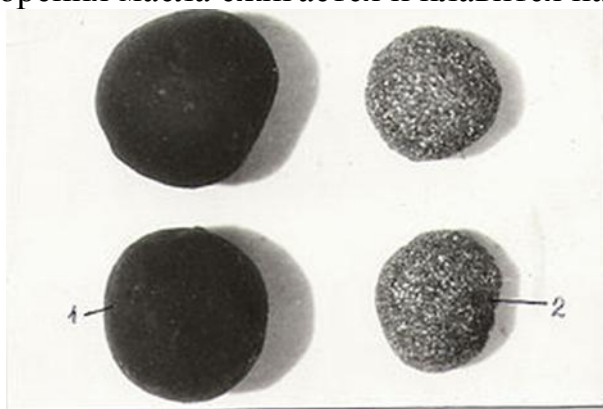
Рис. 15.4. Адгезионноеобогащение золота: а –исходные углемаляные гранулы; б - золотонаполненные гранулы
