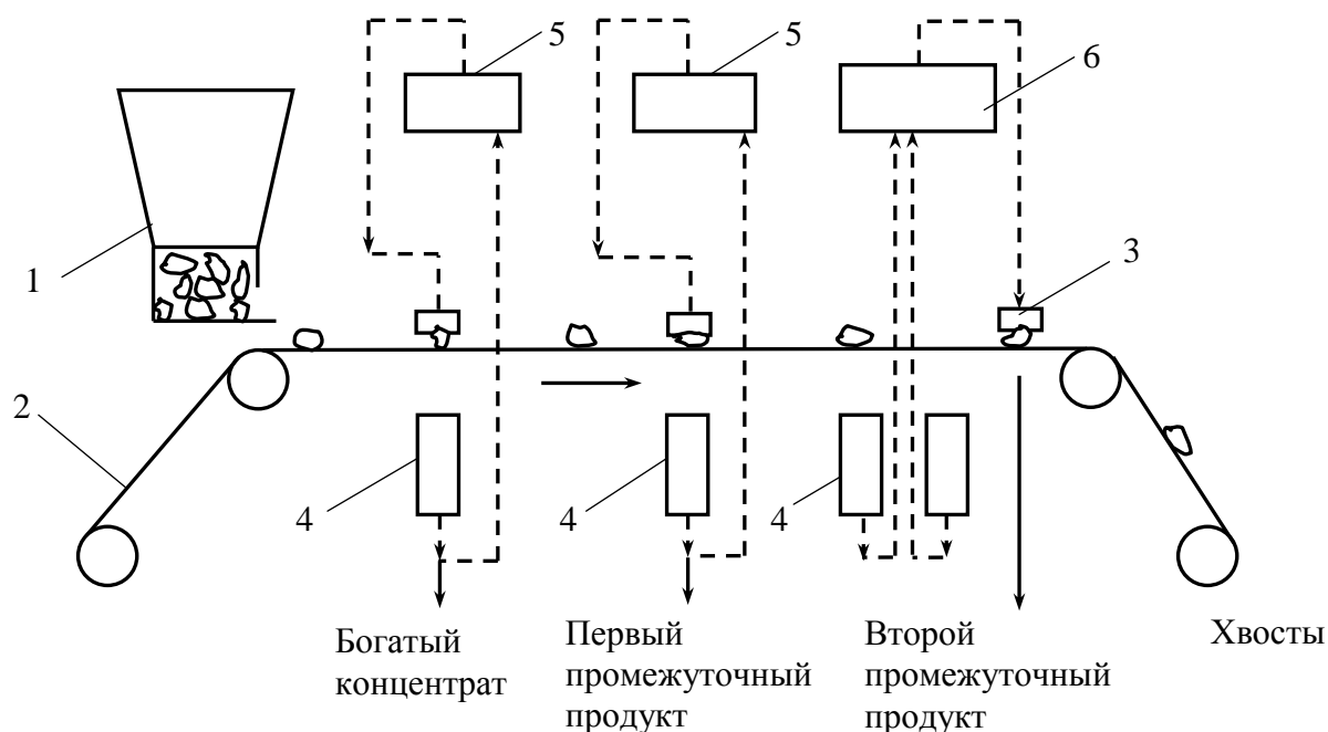
Рис. 4.1. Схема авторадиметрического сепаратора:
