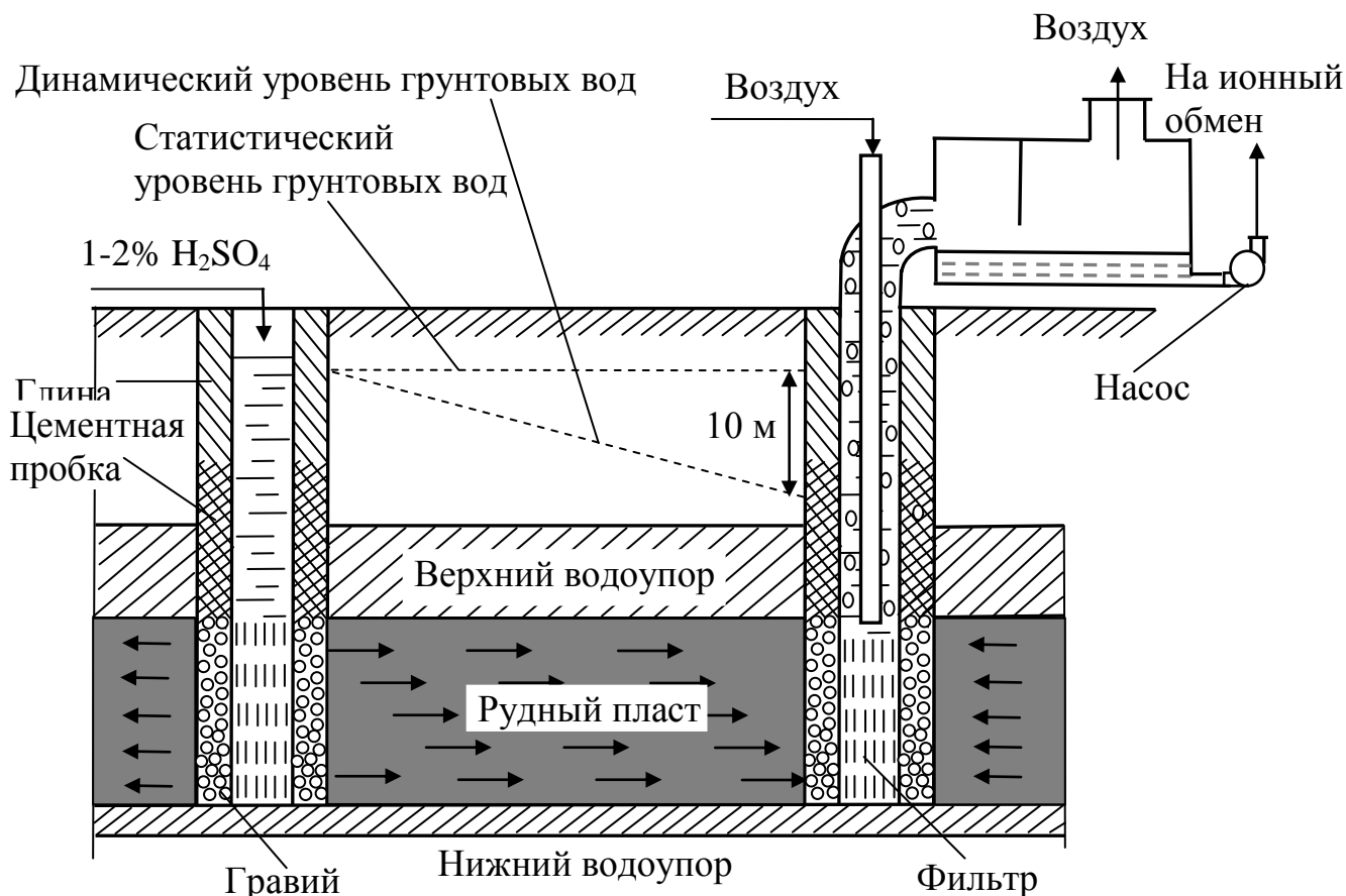
Рис.17.6. Схема подземного выщелачивания урана
