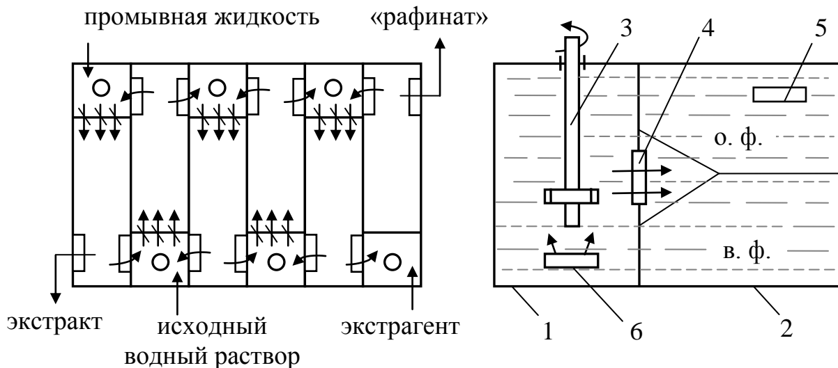
Рис. 18.9. План и поперечный разрез экстрактора «ящичного типа»: 1 – смесительная камера; 2 – отстойная камера; 3 – турбинная мешалка; 4 – жалюзийное окно; 5 – перелив органической фазы; 6 – перелив водной фазы.
