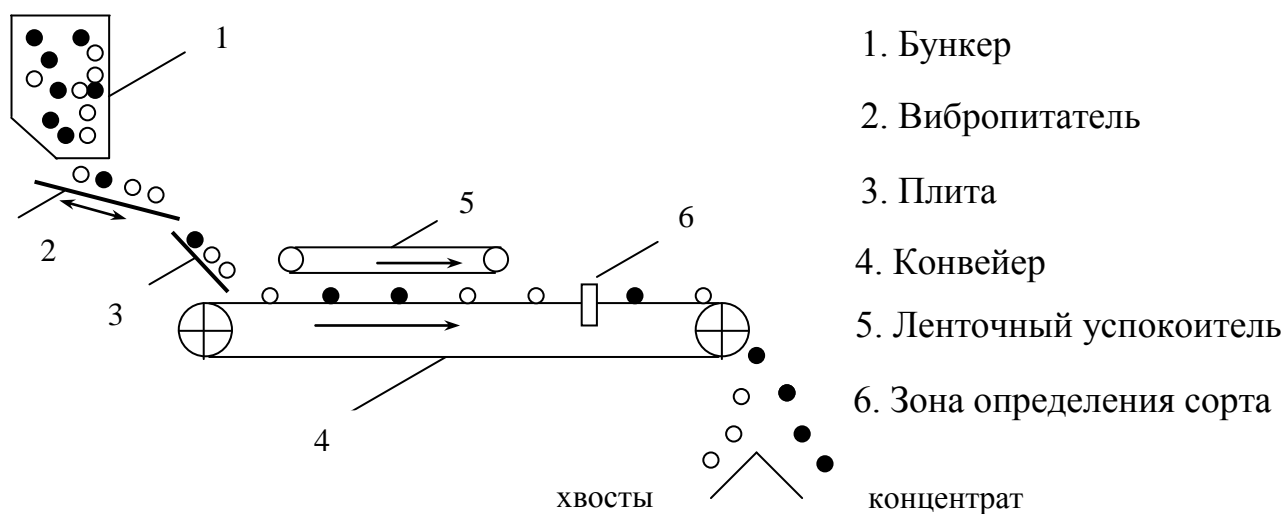
Рис. 3.4. Статистическое формирование плоскокусовой подачи материала
