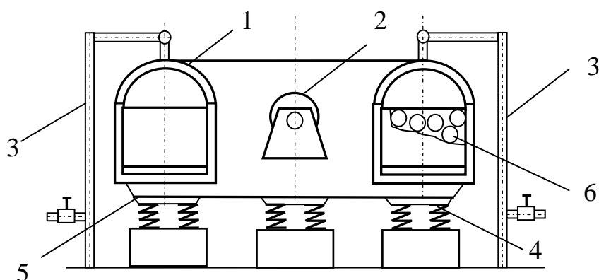
Рис. 12.4. Схема дезинтегратора ДВ-1:
