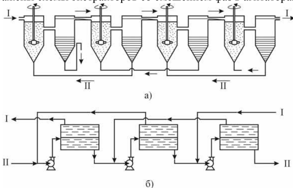
Рис. 18.7. Горизонтальные смесительно-отстойные экстракторы со смешиванием фаз в агитаторах (а) и в насосах (б):
