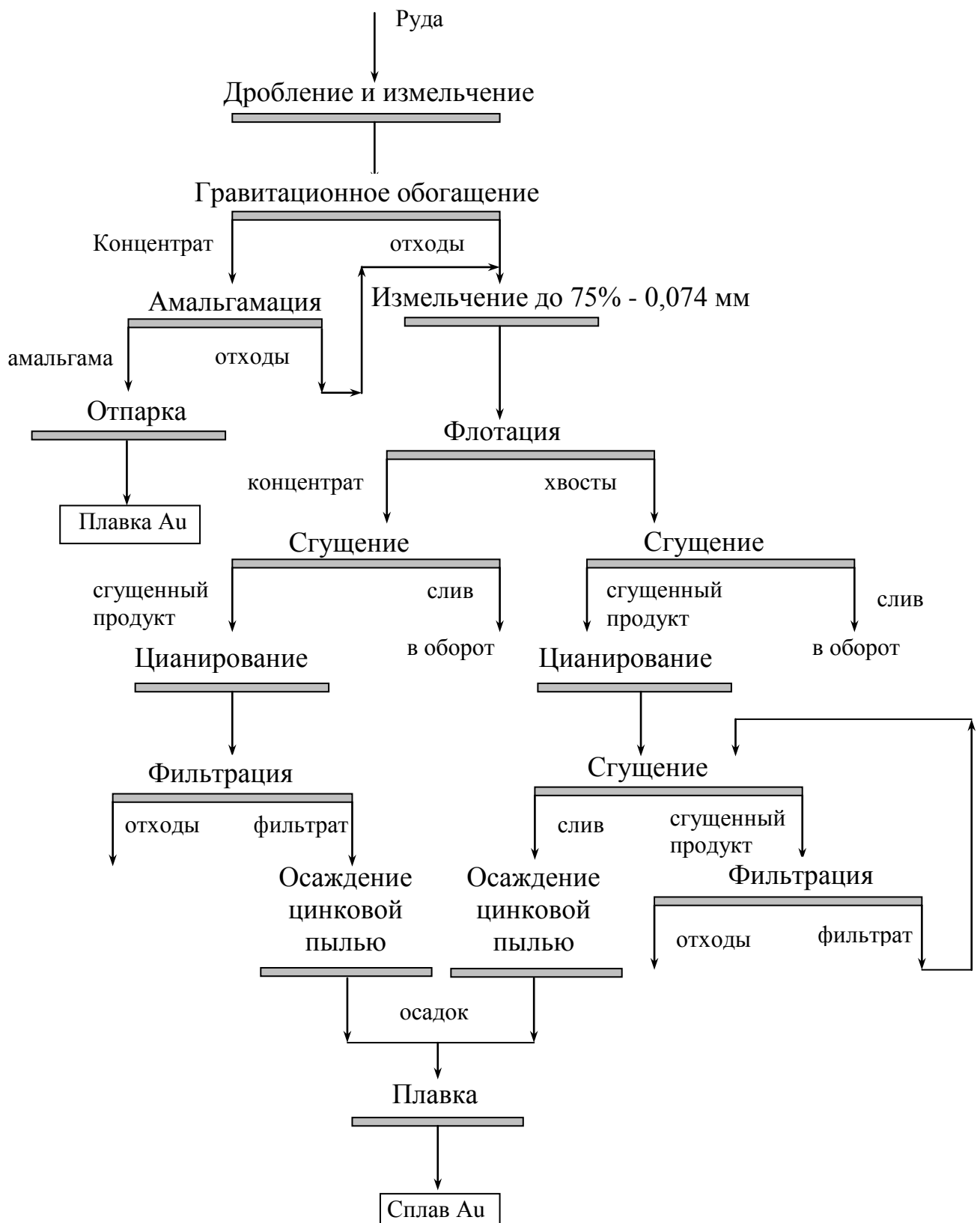
Рис. 20.3. Схема извлечения золота из коренной руды
