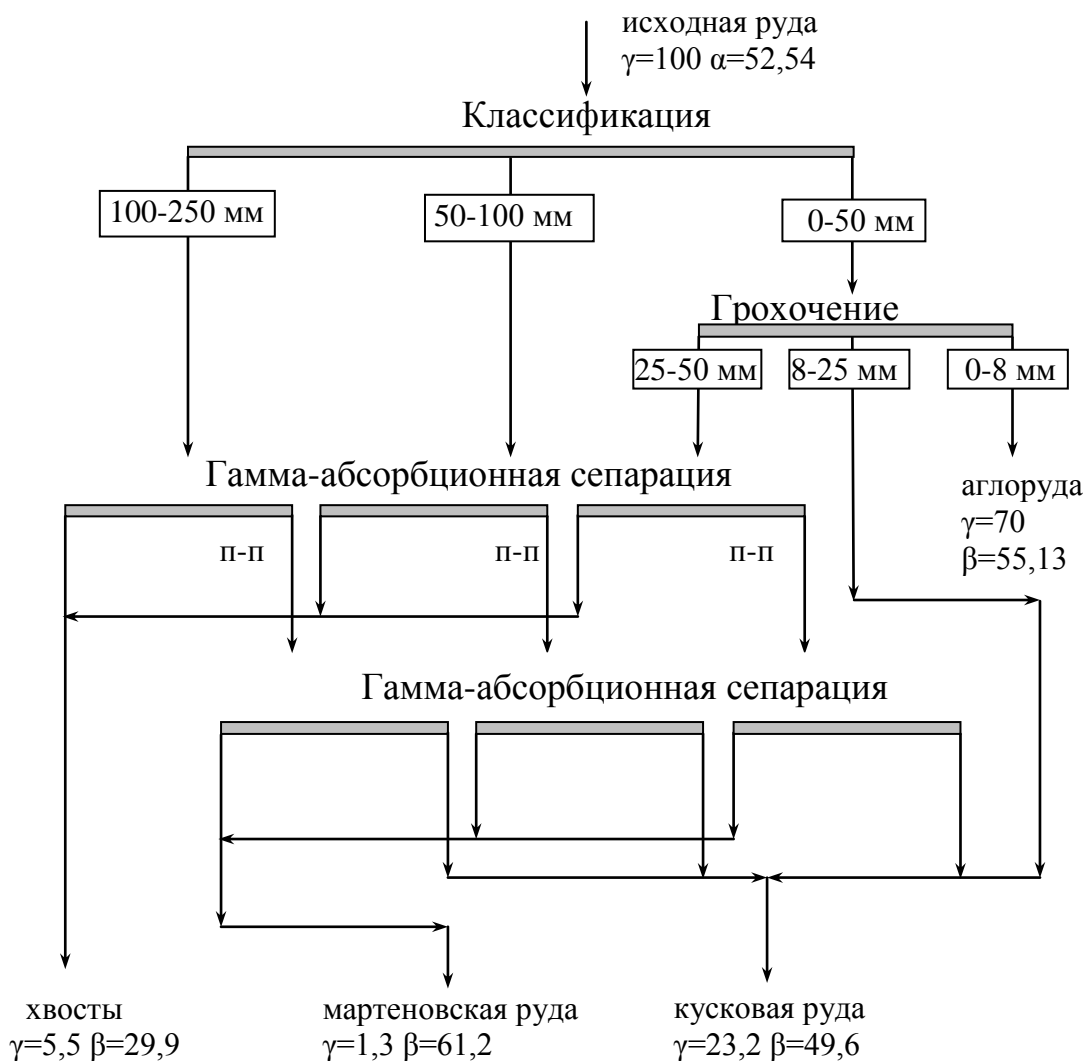
Рис. 6.5. Схема радиометрической сепарации железных руд
