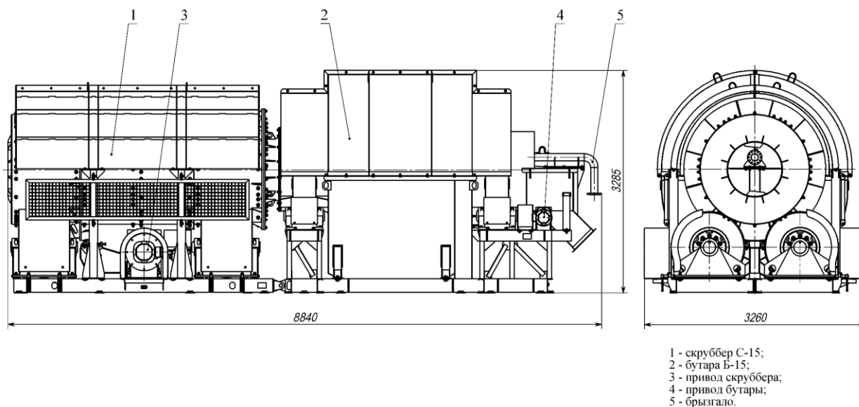
Рис. 11.4. Промывочно-сортировочный комплекс ПСК-80
