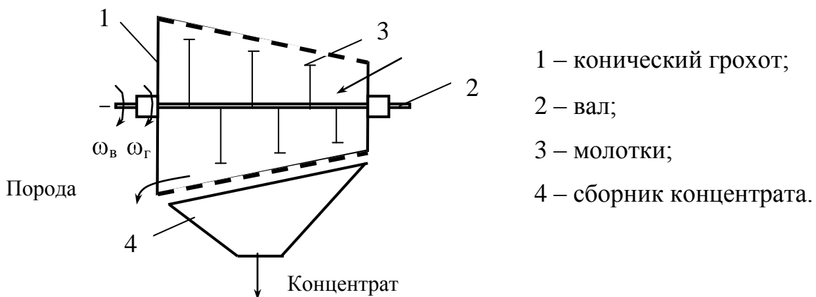
Рис. 10.1. Дробилка ударного действия
