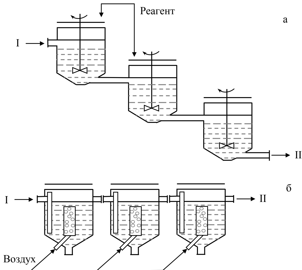
Рис. 17.2. Каскады выщелачивания: а) – из трех аппаратов с механическим перемешиванием; б) – из трех пачуков
