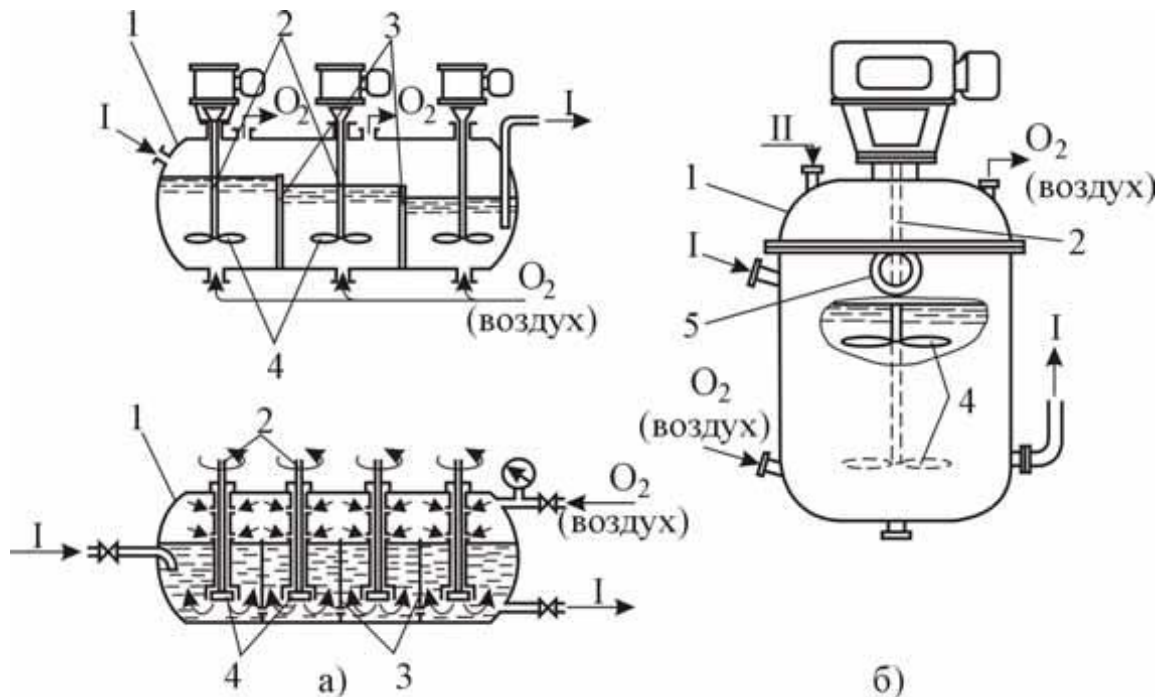
Рис. 17.3. Горизонтальные многосекционные (а) и вертикальный (б) автоклавы с механическим перемешиванием пульпы, работающие под повышенным давлением кислорода или воздуха: I – пульпа, II – выщелачивающий реагент; 1 – корпус; 2 – валы мешалок; 3 – перегородки; 4 – пропеллерные мешалки; 5 – смотровое окно
