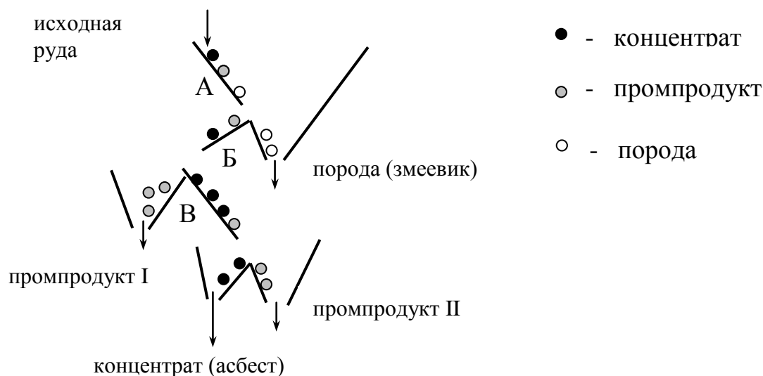
Рис. 8.5. Сепаратор для обогащения по трению «Горка»
