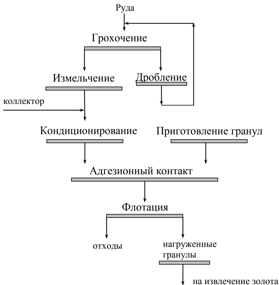
Рис. 15.5. Процесс CGA компании "British oil and minerals" и "Davy McKee"
