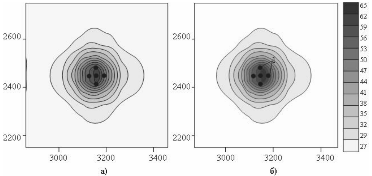
Рис. 5. Распределение температуры шахтных вод ( ^{\circ}\text{C} – оттенки серого цвета) вблизи (расстояния в метрах) куста «теплых» скважин 1: а, б – соответственно к концу отопительного и летнего периода
