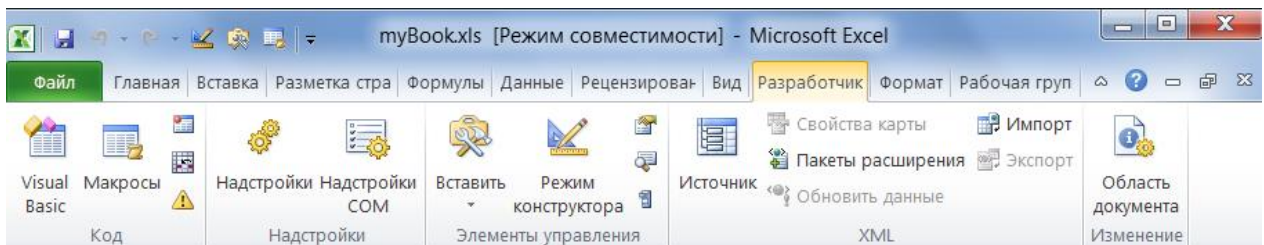
Рисунок 6.2 – Вкладка «Разработчик»
