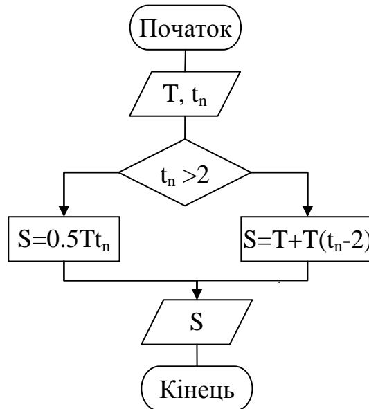
Рисунок 1.2. Приклад алгоритму розгалужених обчислень
