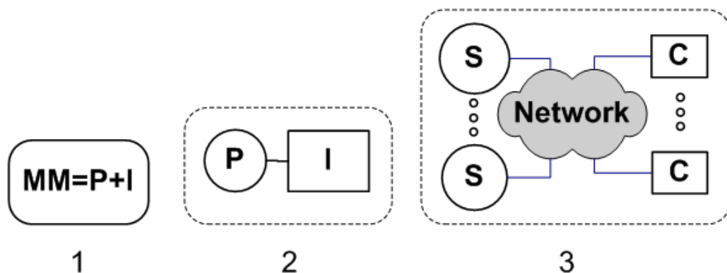
Рис. 5. – Схема развития интегрированных моделирующих сред: 1 – монокодовый этап, в котором монокодовая модель (ММ) представляется как неразрывное единство процессорной части (P) и интерфейсной (I); 2 – дикодовый этап, наиболее характерный для современной вычислительной техники, привел к существенному разделению собственно вычислений (P) и интерфейса (I); 3 – гиперкодовый этап характерен для формирующейся в настоящее время сетевой среды, в которой не просто разделенными, а распределенными структурно и пространственно оказываются вычислительные серверные компоненты (S) и интерфейсные клиентские (C).
