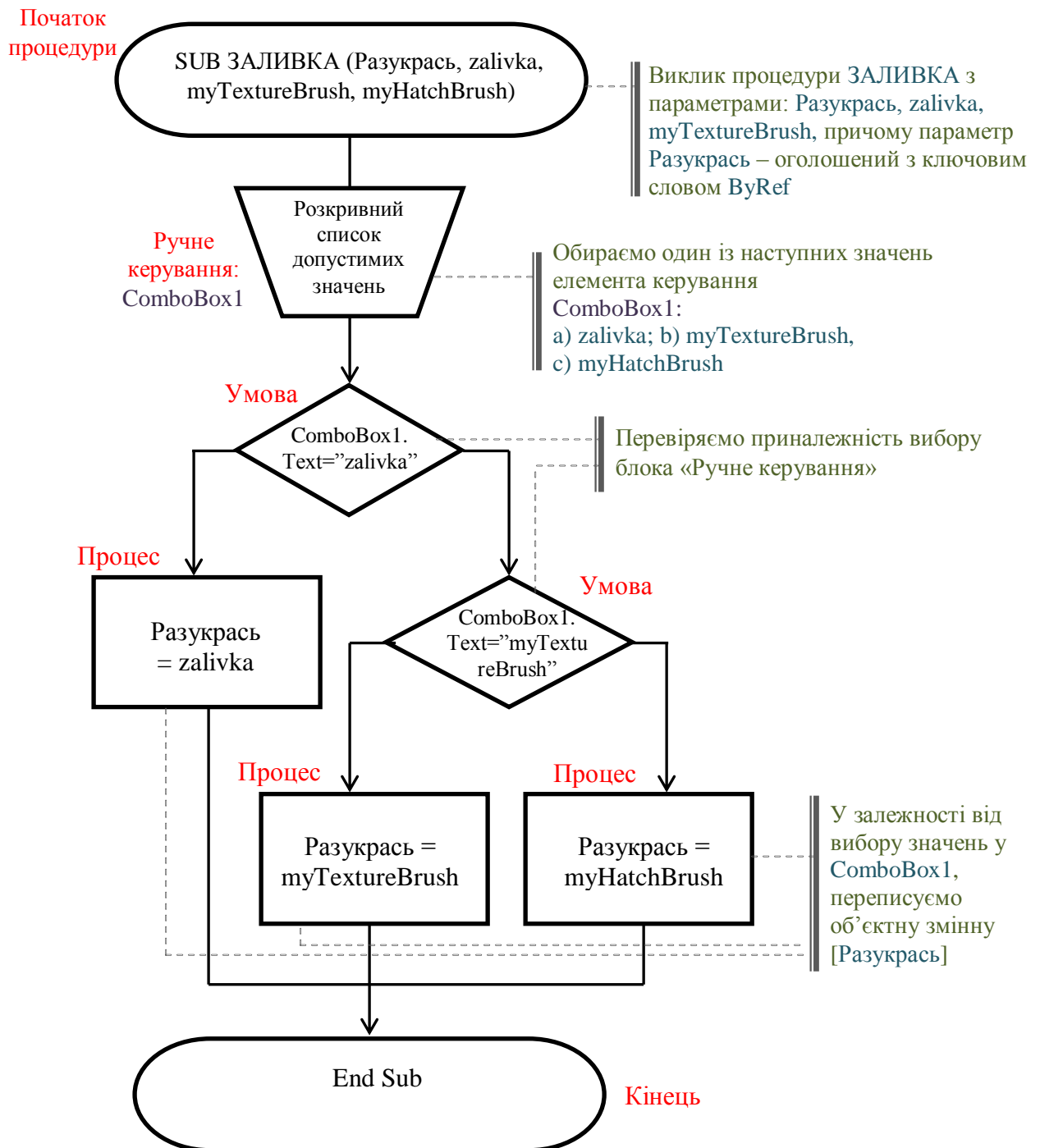
Рисунок 4.13 – Блок-схема процедури «Заливка» моделі «Графіка»
