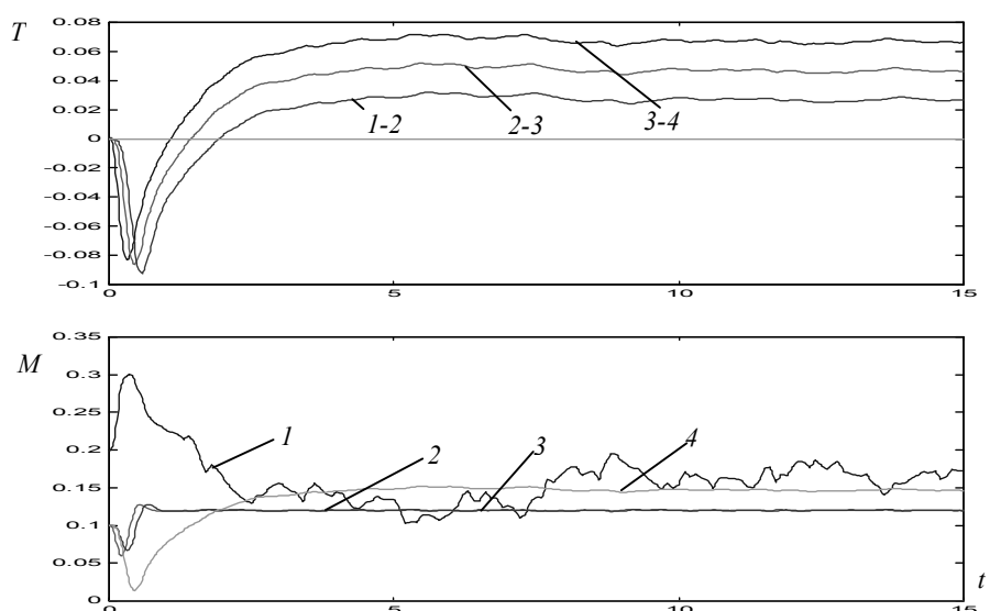
Рисунок 3 – Реакция моментов главных приводов M и межклетевых натяжений T на случайное изменение толщины подката 4-х клетевых прокатного стана
