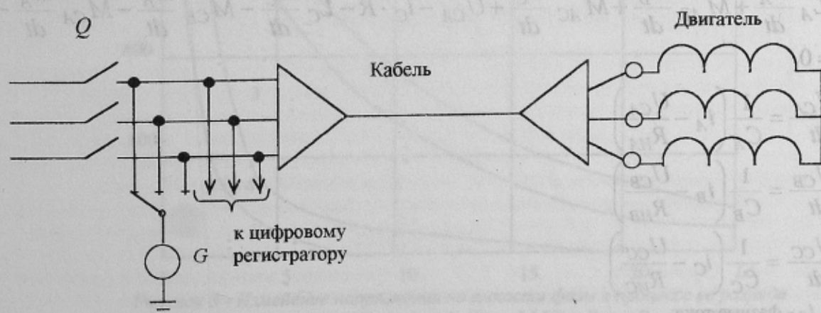
Рисунок 1- Схема проведения измерений при диагностике присоединения
