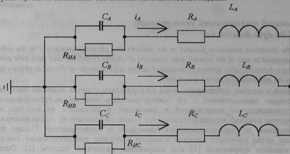
Рисунок 2- Схема замещения присоединения кабель-двигатель.
