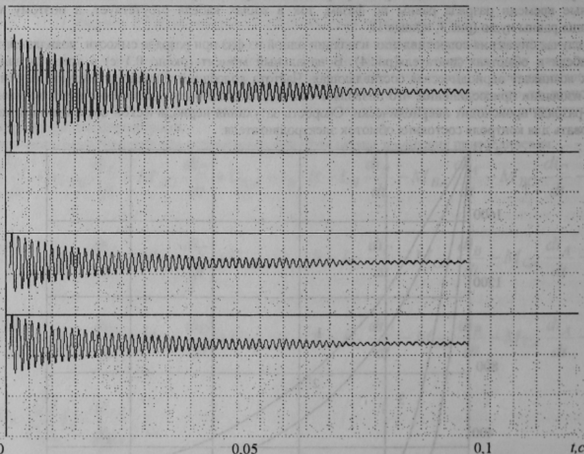
Рисунок 4 - Изменение токов фаз А, В и С в начальный период разряда емкостей при снижении сопротивления изоляции в фазе А
