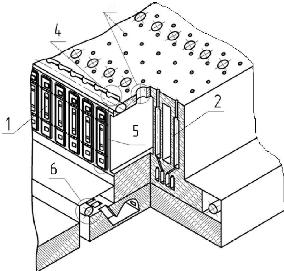
- Рисунок 1 -. Выбросоопасные зоны и элементы коксовой батареи: 1 - двери коксовых печей; 2 - обогревательные простенки; 3 - загрузочные люки и смотровые шахточки; 4 - стояки, газосборники, газоотводящие люки; 5 - элементы придверной зоны; 6 - элементы газоподводящей арматуры
