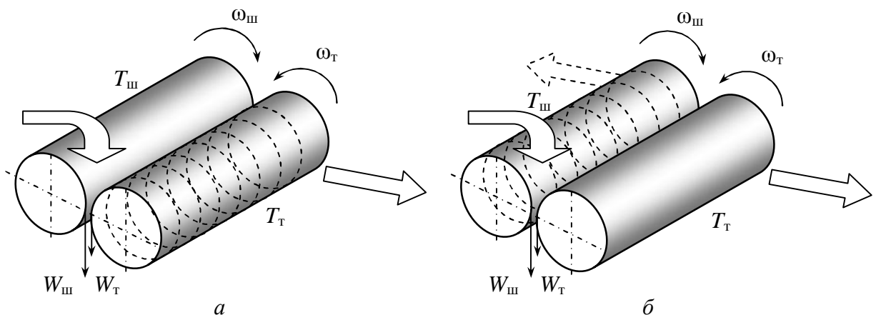
Рис. 1. Схема безперервного вальцювання з відбиранням стрічки матеріалу з тихохідного (а) і зі швидкохідного (б) валка: \omega_{ш} , \omega_{т} – кутова швидкість швидко- і тихохідного валка; W_{ш} , W_{т} – лінійна швидкість швидко- і тихохідного валка; T_{ш} , T_{т} – температура швидко- і тихохідного валка (стрілками показано варіанти завантаження й знімання композиції)
