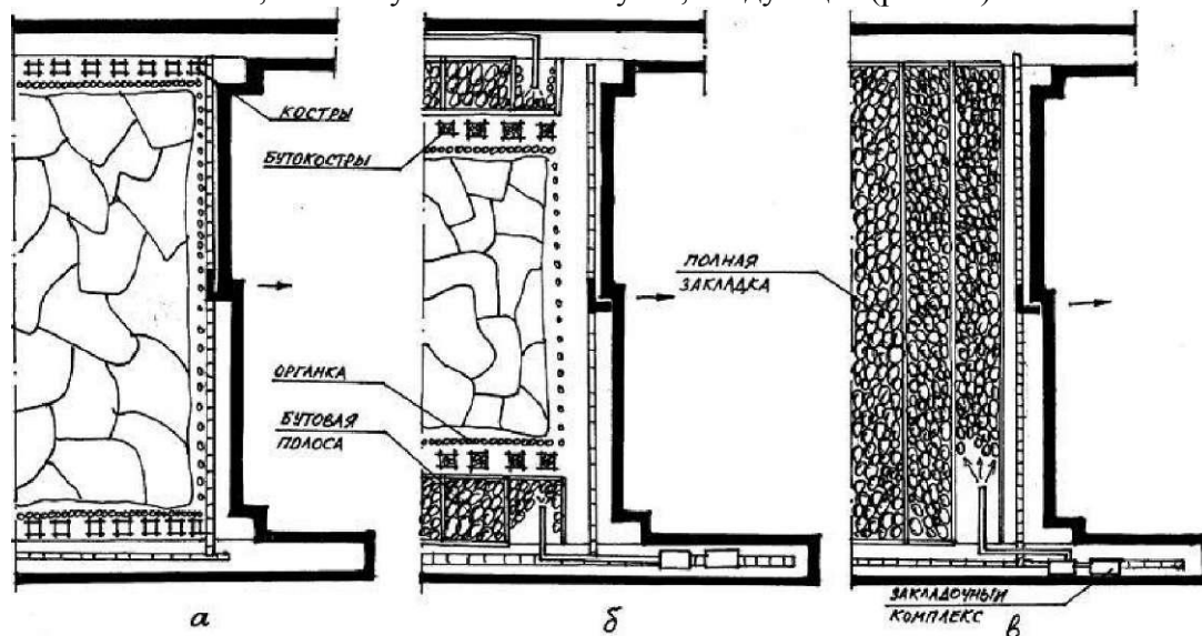
Рис. 4 - Технологические схемы крепления в очистном забое: а - используемая на шахте «Украина»; б - рекомендованная к применению (вариант 1); в - рекомендованная к применению (вариант 2)
