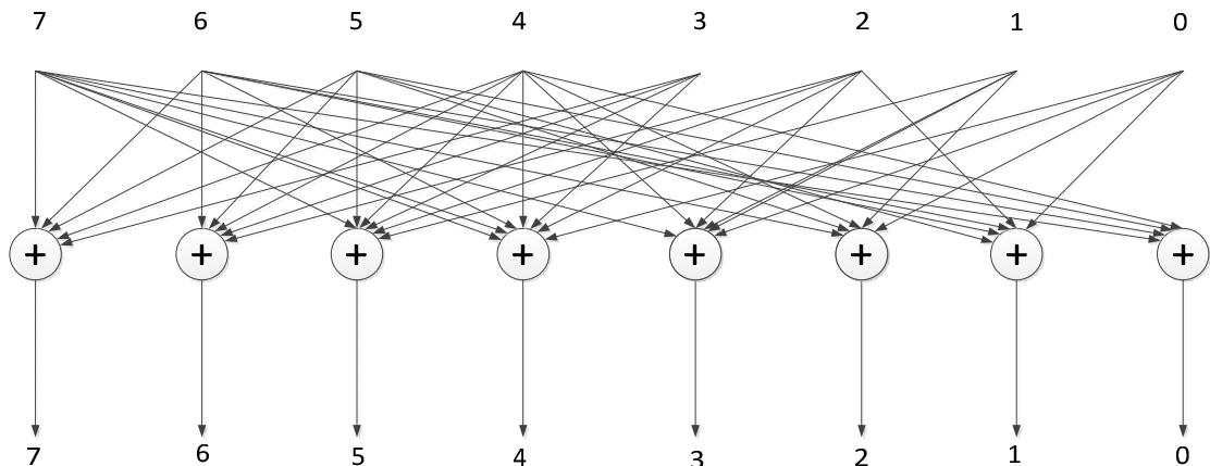
Рисунок 2 - Реализация умножителя на константу для псевдопеременной X^3 на элементах двоичной логики
