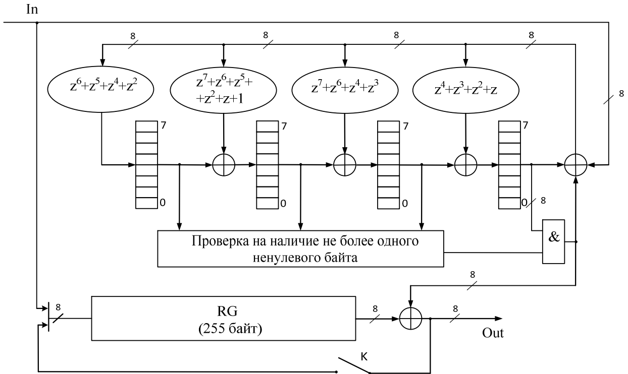
Рисунок 1 - Декодер (255, 251) кода Рида-Соломона, исправляющего двойные ошибочные байты
