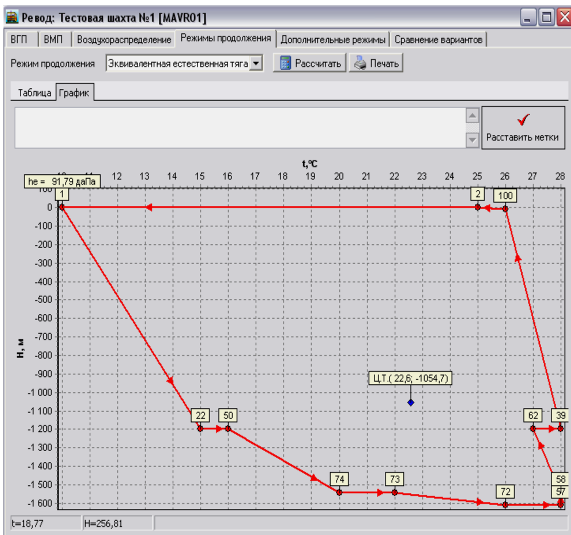
Рис.1. Многоугольник эквивалентной естественной тяги (пример 1)
