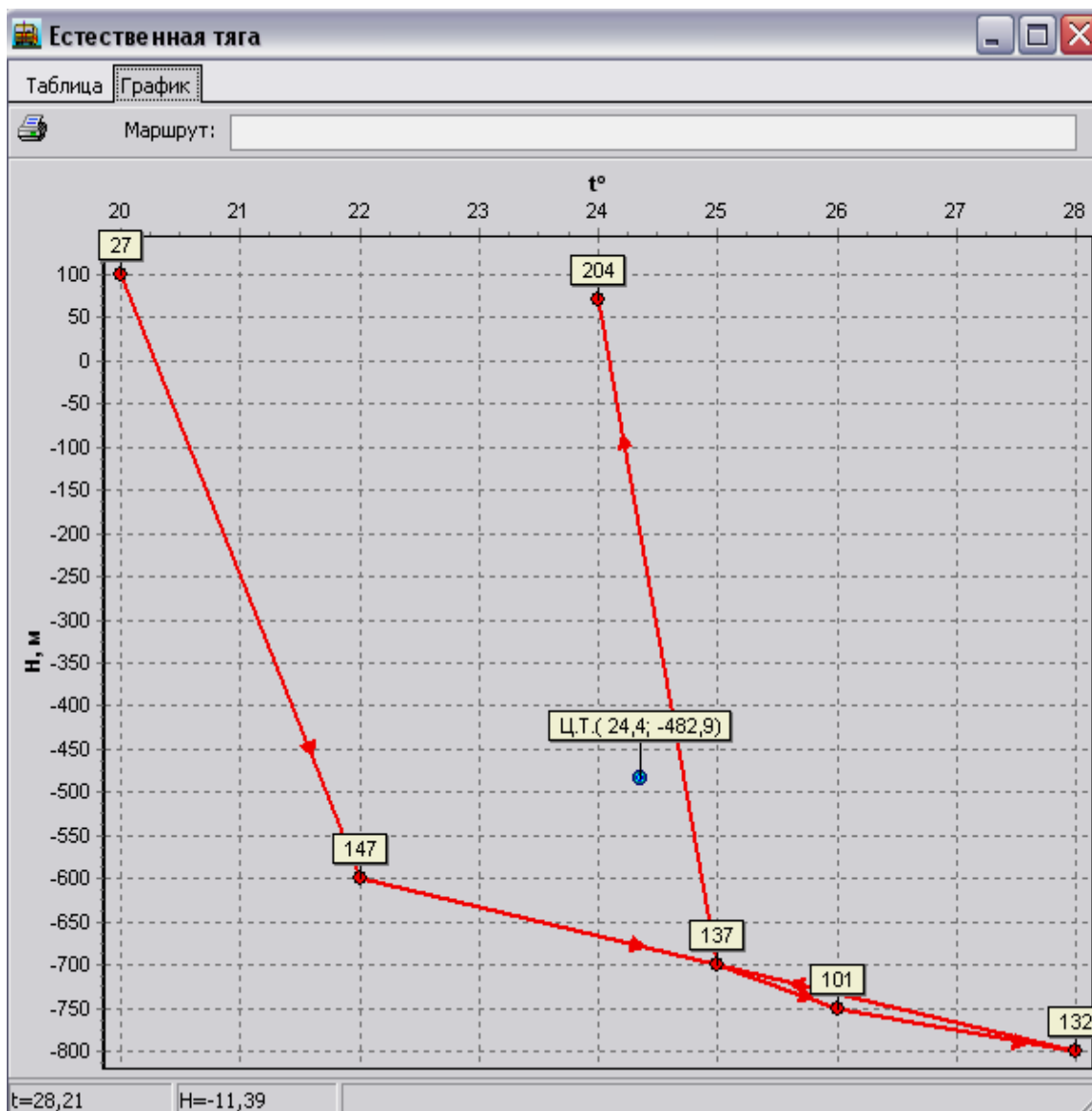
Рис.2. Многоугольник эквивалентной естественной тяги (пример 2)
