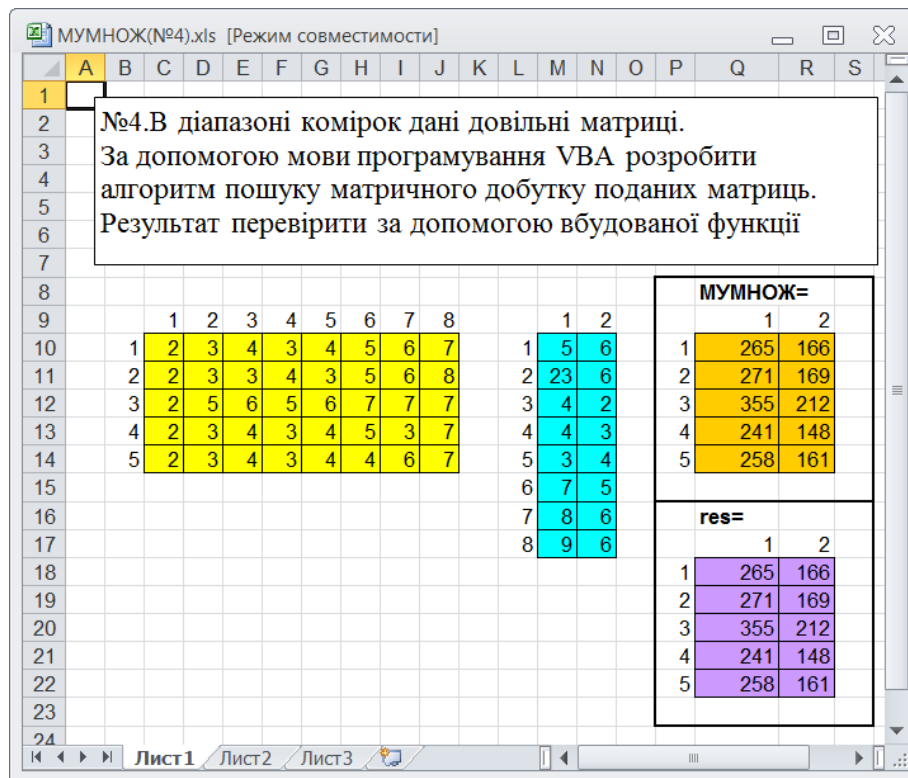
Рисунок 6.13 – Робочий аркуш
