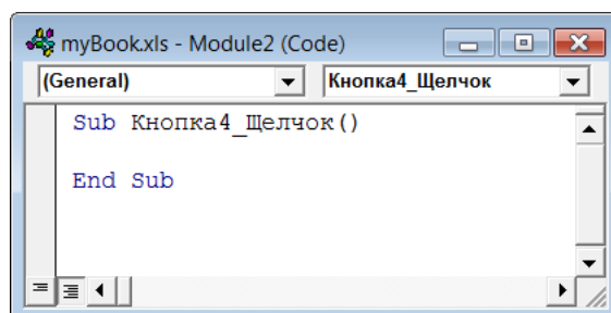
Рисунок 6.8 – Процедура макросу
