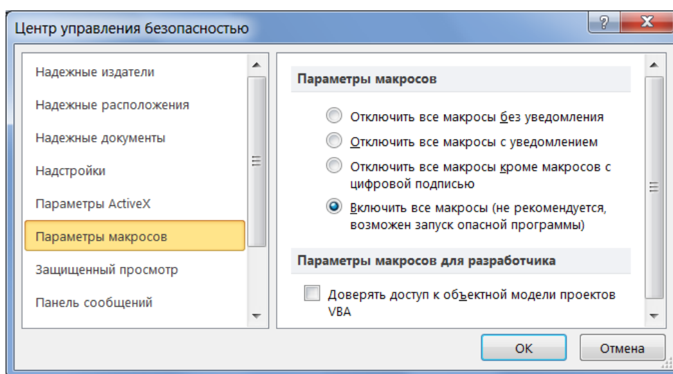
Рисунок 6.3 – Параметры макросів
