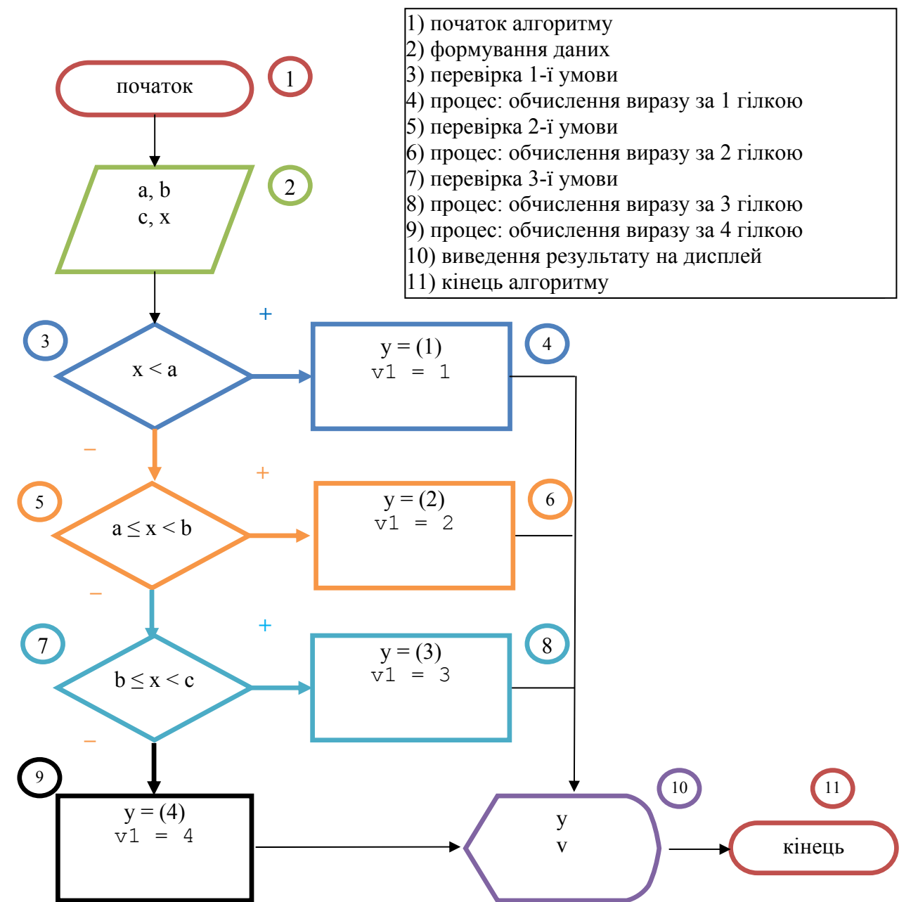
Принципова блок-схема алгоритму
