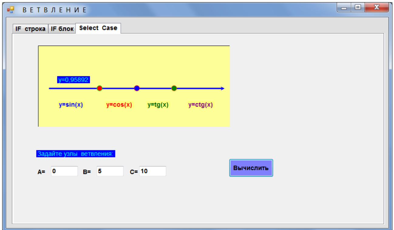
Рисунок 3.3 – Форма задачі «Алгоритм розгалуження 4 гілки»
