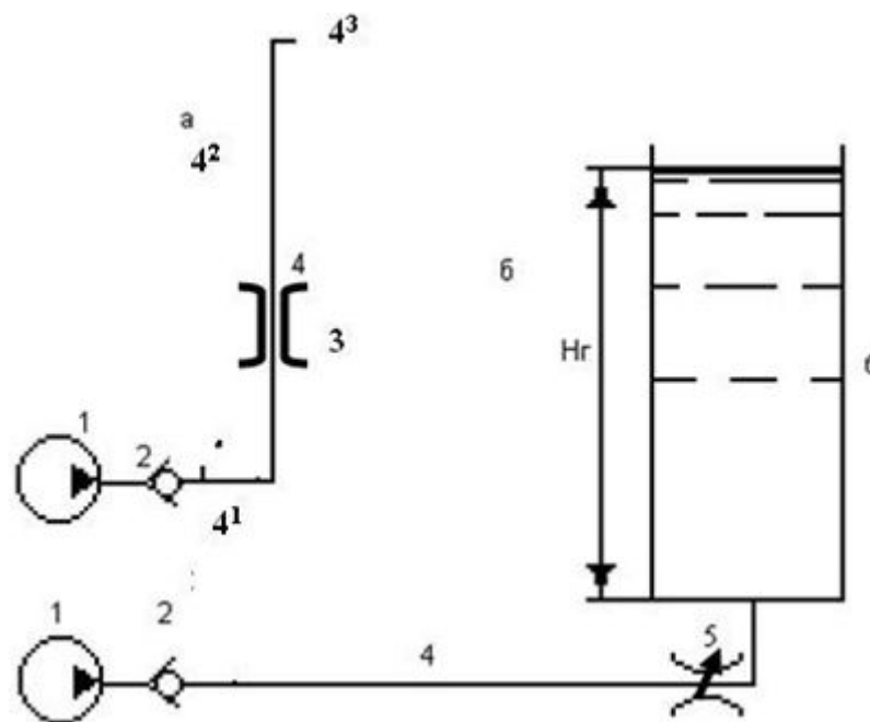
Рис. 1 – Водоотливная установка: а – схема; б – расчетная модель; 1 – насос, 2 – обратный клапан, 3 – функциональный дроссель, 4 – трубопровод (41 – горизонтальный участок, 42 – вертикальный участок 43 – участок на поверхности), 5 – переменное гидравлическое сопротивление трубопровода, 6 – резервуар глубиной, равной геометрической высоте трубопровода
