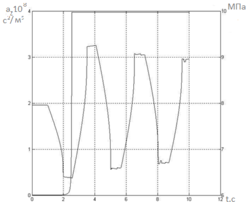
Рис. 3 – Расчет гидравлического удара в трубопроводе водоотливной установки
