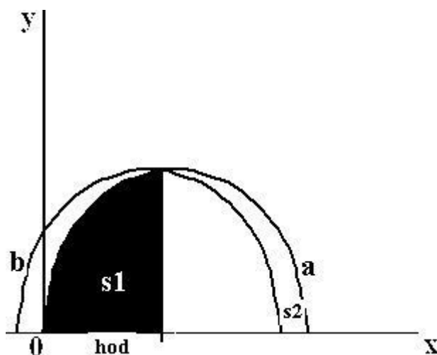
Рис. 4 – Расчетная схема задвижки в процессе закрытия: а – корпус; б – затвор
